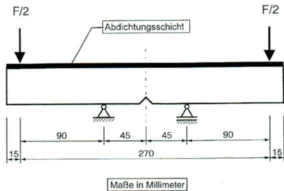
Abbildung 1: Belastungsanordnung
