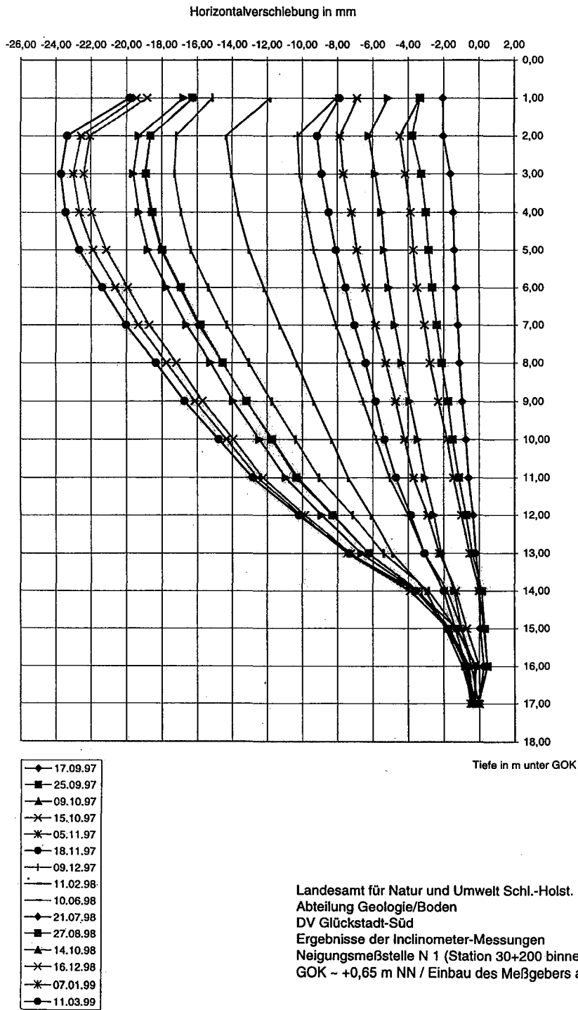
Abb. B 17: Tiefenbezogene Darstellung der Horizontalverschiebungen bei Dkm 30 + 200 Glückstadt-Süd
