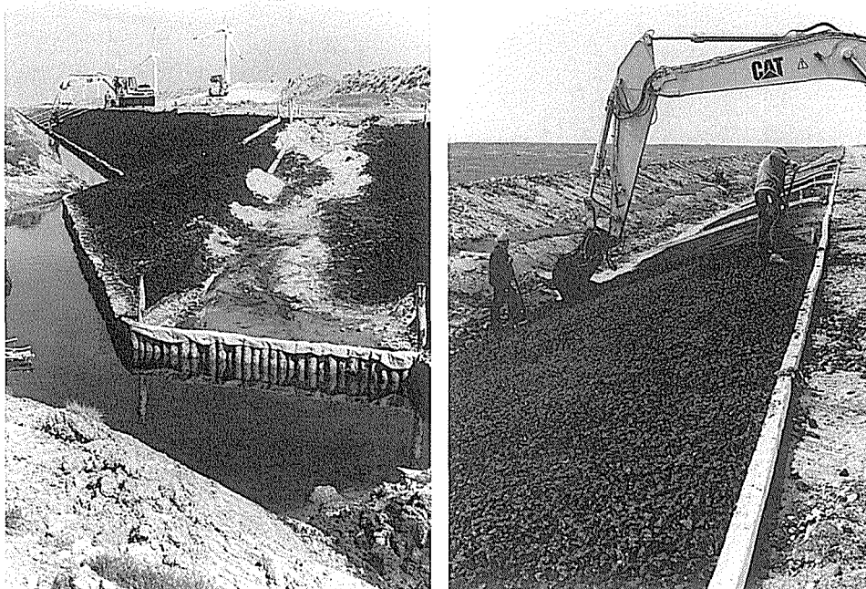
Abb. G 50b+c: Deichverstärkung Friedrich-Wilhelm-Lübke-Koog hinter Vorland 2001/2002: Einbau von Mastixschotter als Fußdeckwerk auf Bitumensand-Filter bis zur Überslaggsicherung
