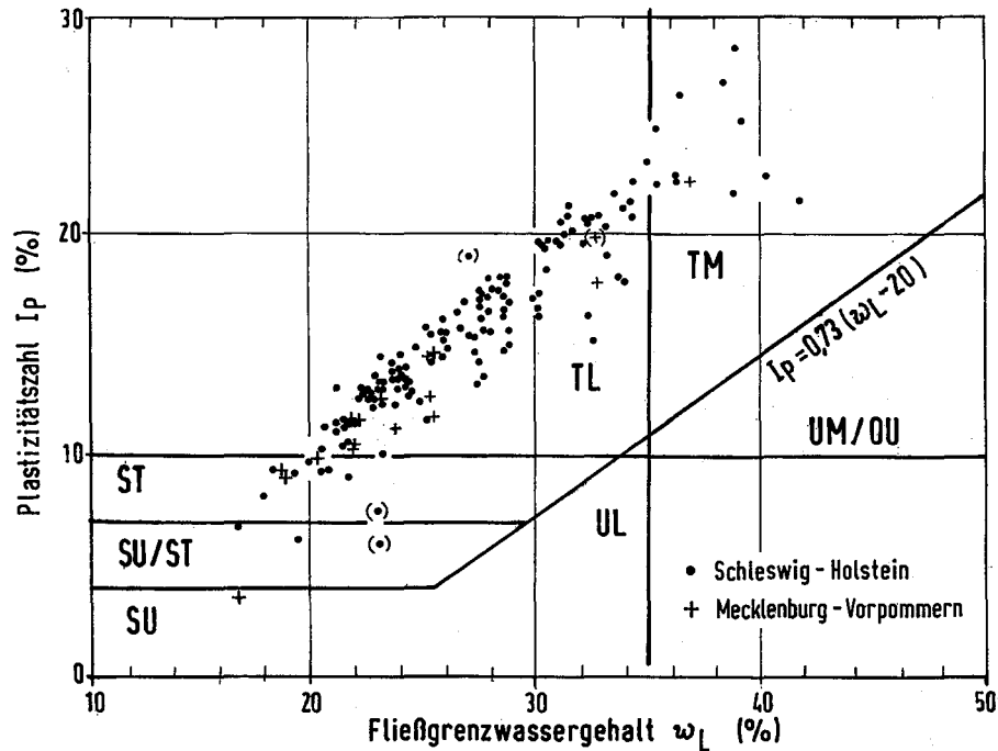
Abb. G 26: Plastizitätskarte von Geschiebeeböden
