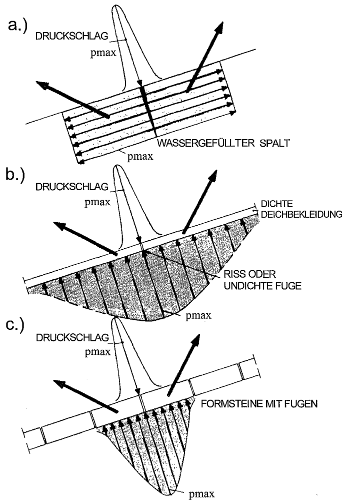
Abb. A 4.2.6: Sprengwirkungen von Druckschlägen auf Risse und Fugen (nach FÜHRBÖTER, 1966)
