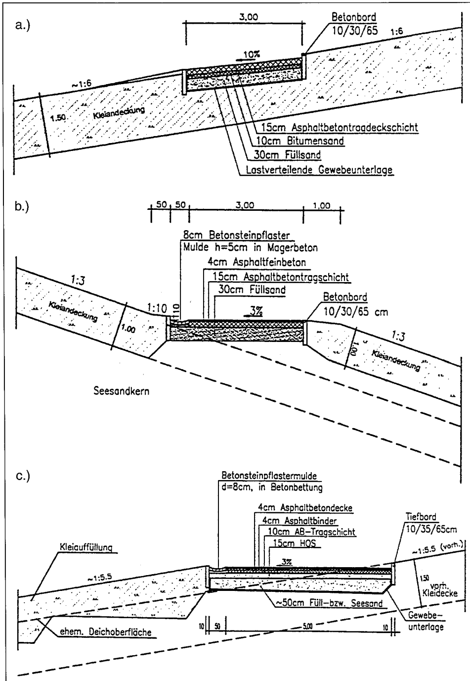
Abb. G 15: Anordnung und Aufbau von Deichrampen an der Nordseeküste a) in der Außenböschung, b) in der Binnenböschung, c) nachträglicher Einbau für ständigen Verkehr in die Außenböschung
