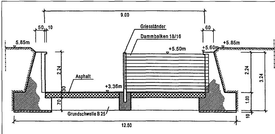
Abb. G 16: Deichstöße Querschnitt
