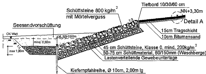
Detail Deckwerk
