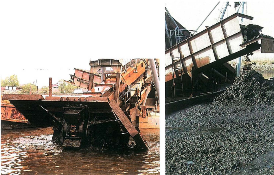
Abb. G 48a + b: Aufnahmegert für Baggergut mit Förderung in Schuten
