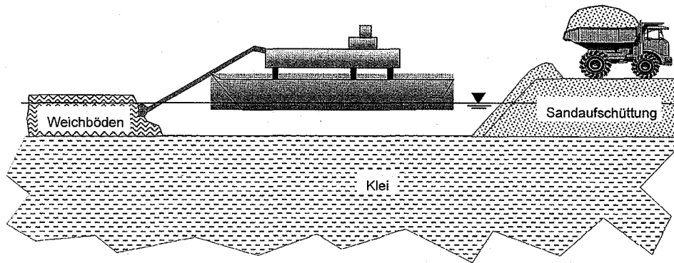
Abb. G 38: Bodenaustausch im Nassbaggerverfahren
