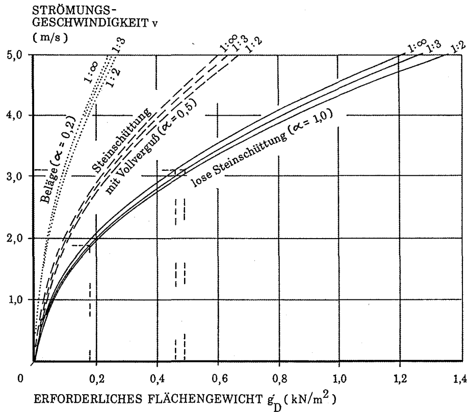
Abb. A 5.11: Erforderliches Flächengewicht von gebundenen Böschungs- und Sohlaukleidungen (durchlässig bei einer Stabilität gegen Abheben von n_z = 1,2 in Abhängigkeit von der Überströmung [bei Schublagerung])
