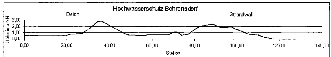
Beispiel 20: Deich mit vorgelagertem Strandwall an der Ostseeküste Schleswig-Holsteins
