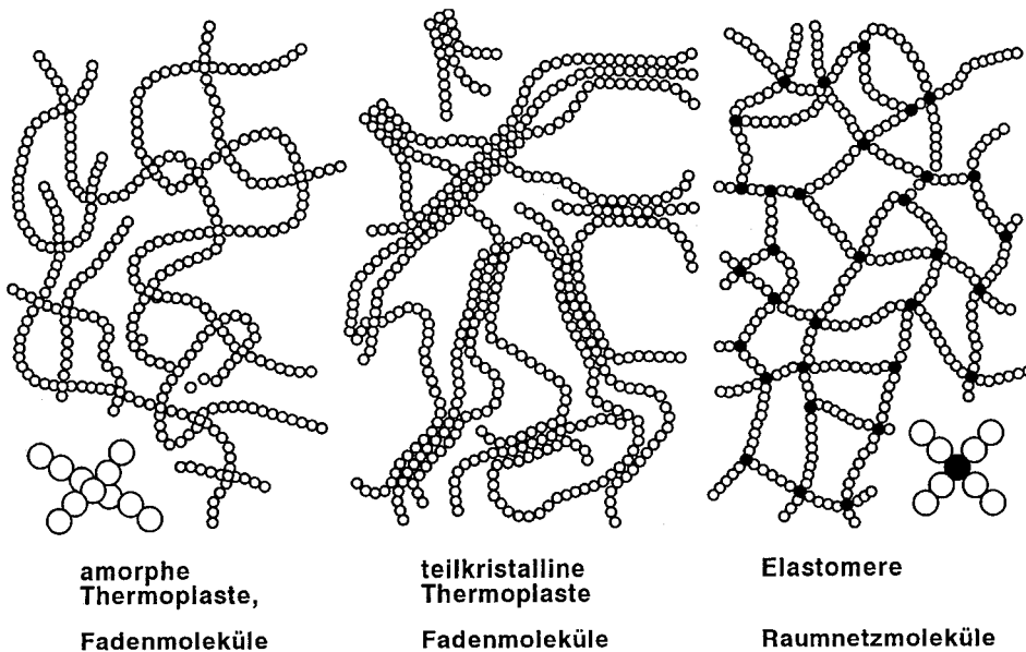
Abb. C 17: Struktur der Kunststoffe (DVWK-Merkblatt, 1992)
