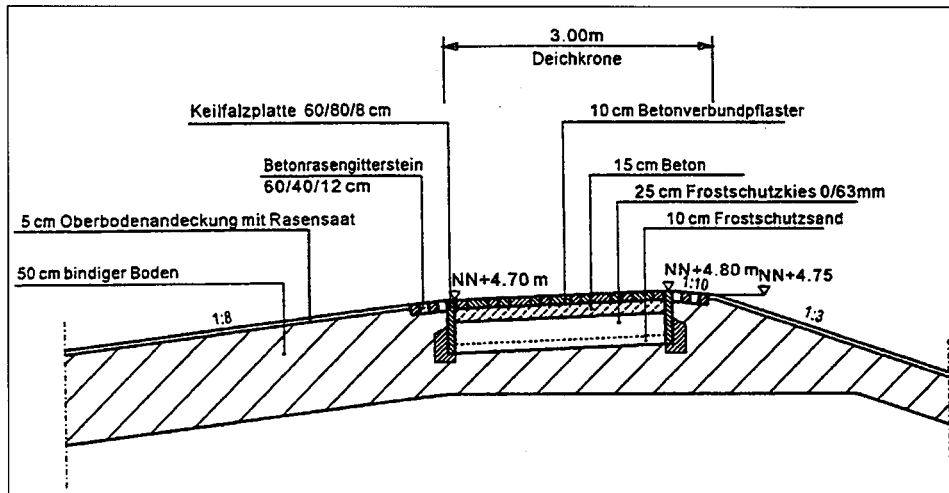
Abb. G 12: Befestigte Deichkrone Grömitz
