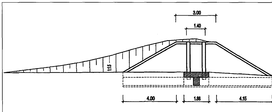
Abb. G 17: Deichstöße Längsschnitt
