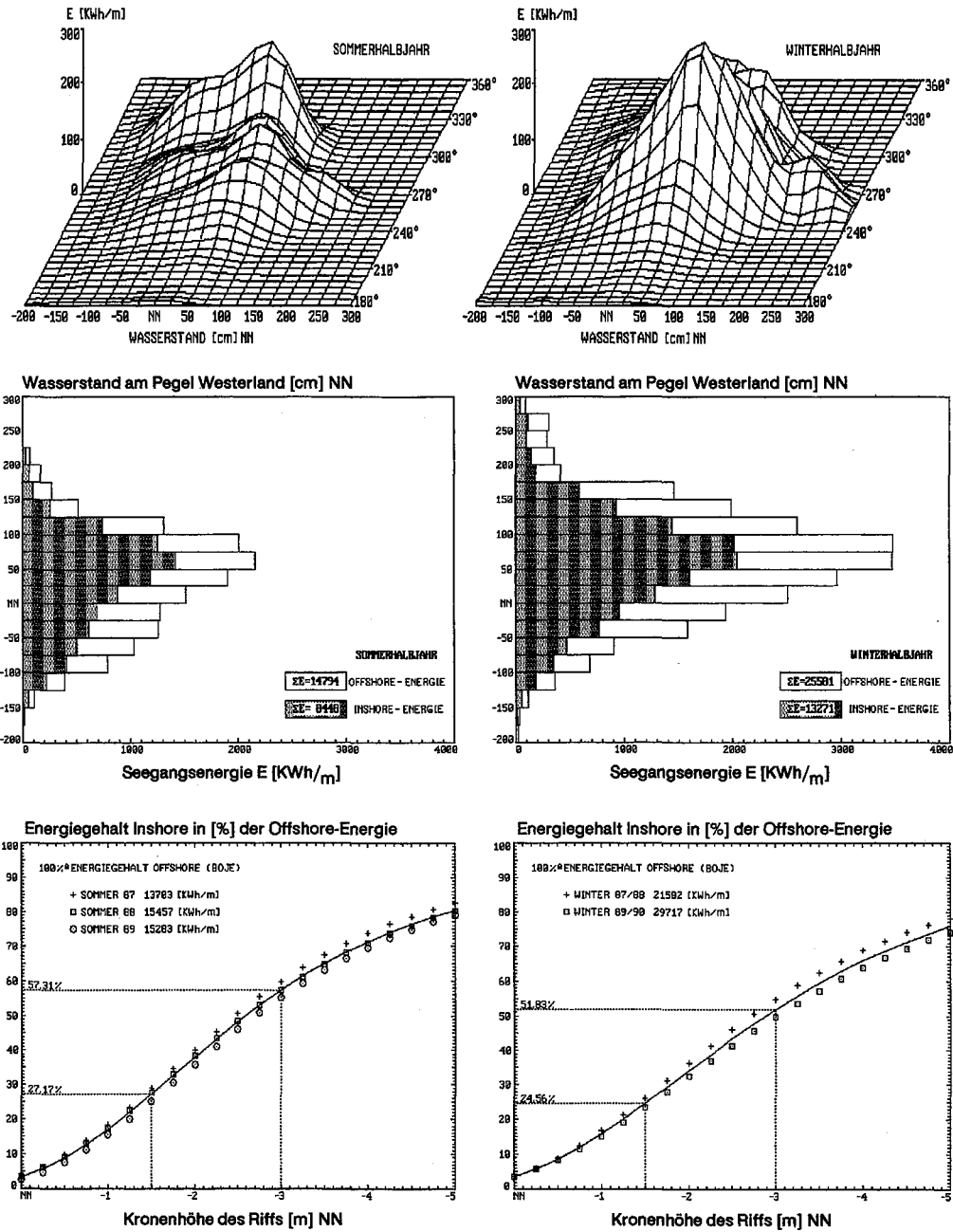
Abb. A 3.38: Vergleichende Darstellung der Offshore- und Inshore Wellenenergien und Einfluss der Kronenlage des Riffs, Beispiel Sylt (STROTMANN u. KOHLHASE, 1991)
