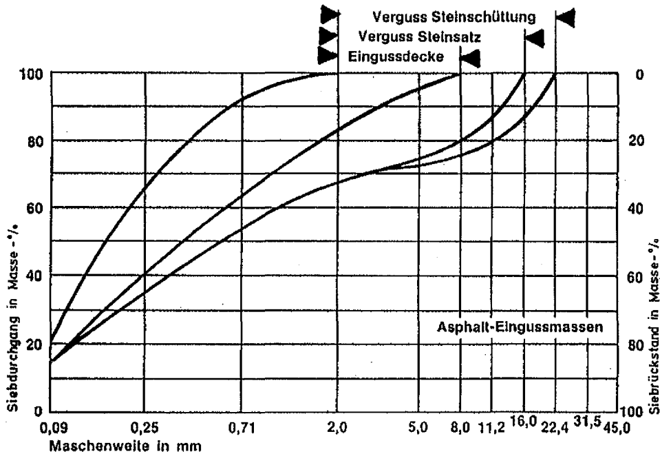
Abb. C 4: Sieblinienbereich für Asphalt-Eingussmassen (Asphaltmastix), (EAAW 83/96)
