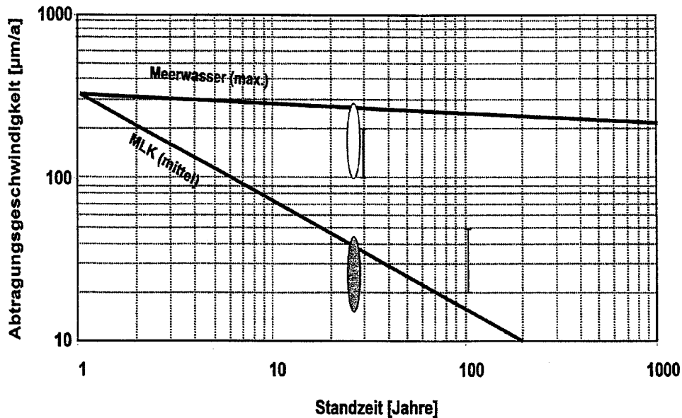
Abb. C 20: Mittlere bzw. maximale Abtragungsgeschwindigkeiten im Mittellandkanal (MLK) und Meerwasser nach (BINDER, 2001)
