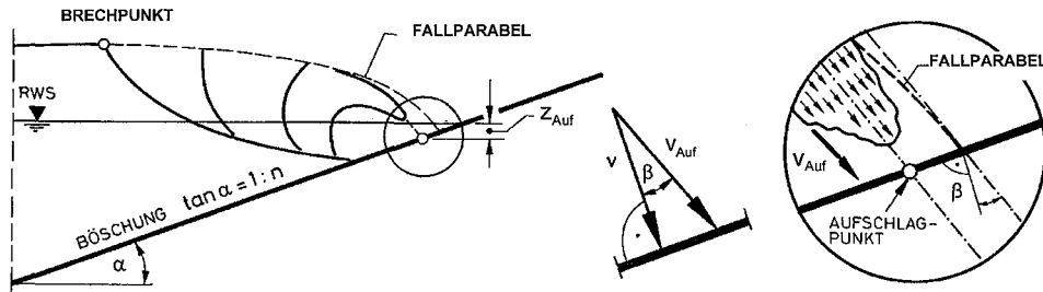
Abb. A 4.2.3: Entstehung der Druckschlagbelastung durch die aufschlagende Brecherzunge von Sturzbrechern (aus FÜHRBÖTER, 1966)
