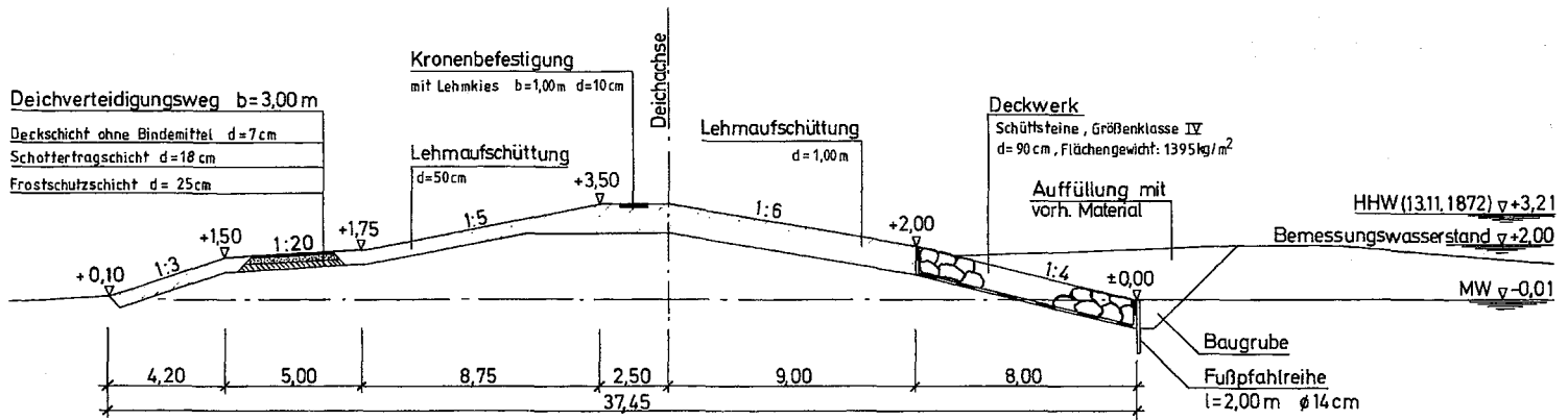
Beispiel 19: sonstiger Deich nördlich der Schleimündung Ostseeküste, Schleswig-Holstein
