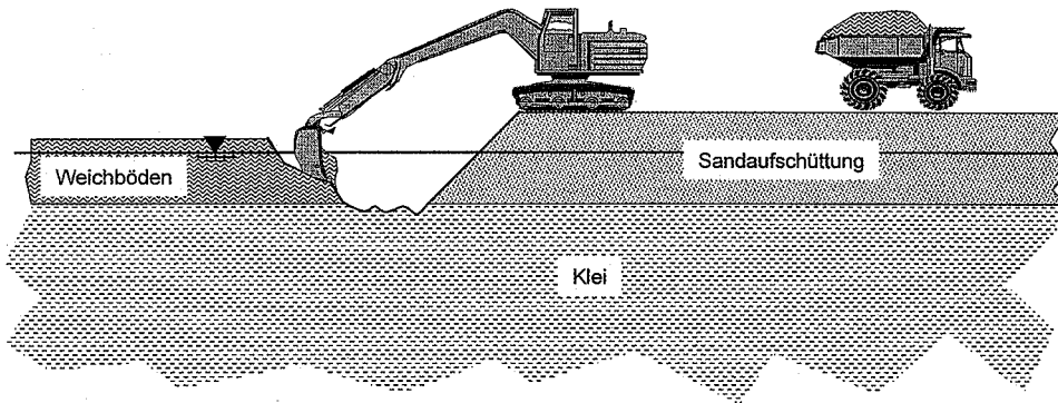
Abb. G 37: Räumung des Weichbodens durch Tieföffelbagger
