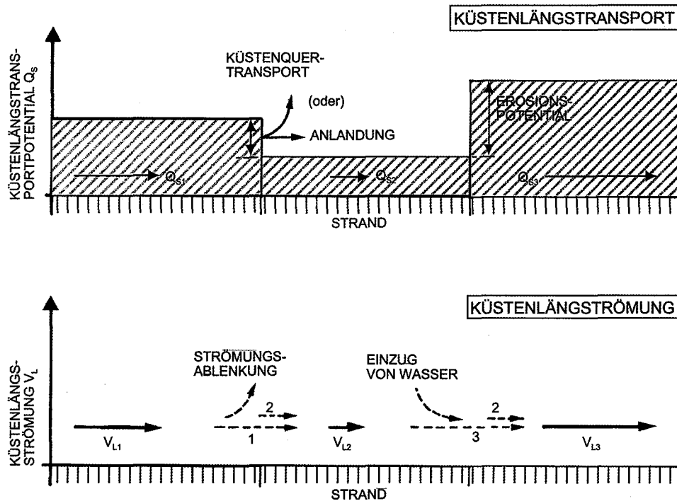
Abb. A 6.9: Schematische Verteilung des Transportpotentials entlang einer Küste infolge Refraktion und Shoaling sowie infolge veränderlichen Verlaufs der Küstenlinie. Die Küstenlängsströmung ist der küstenparallelen Komponente des Energieflusses sowie dem Küstenlängstransportpotential proportional
