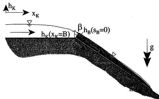
Abb. A 4.2.13: Definition der Strömungsgrößen auf Deichkrone und Deichbinnenböschung
