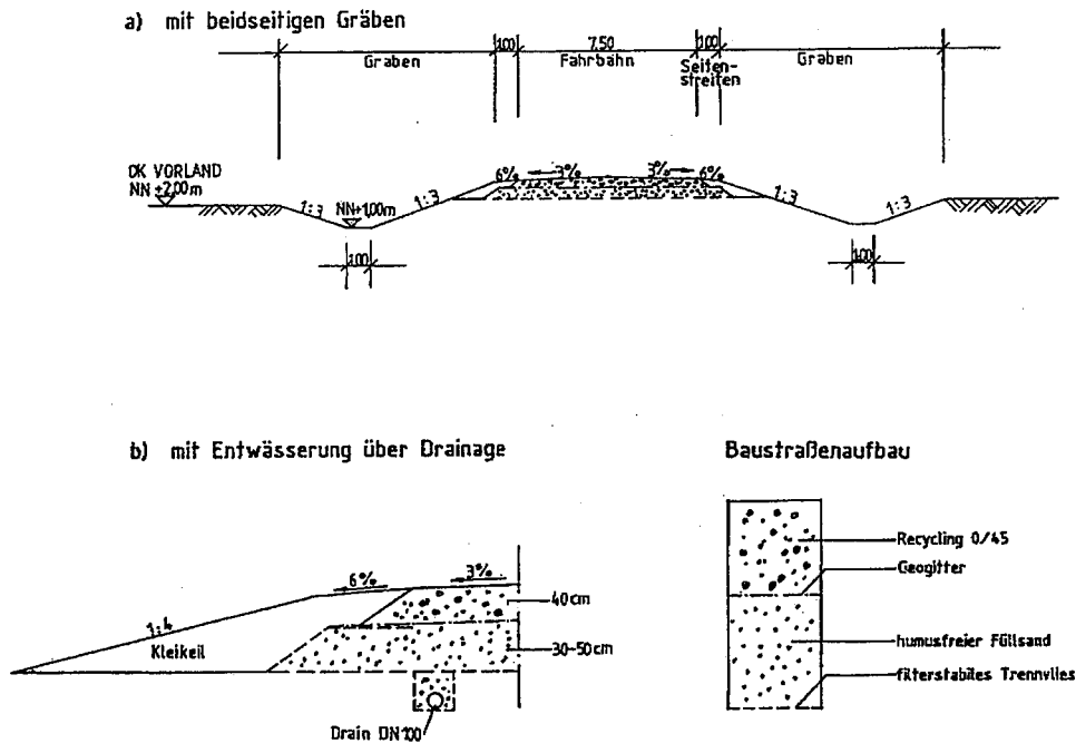
Abb. G 70: Schematischer Querschnitt einer Baustraße in Dithmarschen unter Verwendung eines Geogitters
