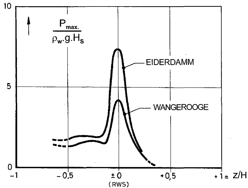
Abb. A 4.2.5: Naturuntersuchungen von GRÜNE (1988) mit Böschungsneigungen 1:n = 1:4: Druckschlaghöhen und -bereiche bei natürlichen Wellenspektren (aus FÜHRBÖTER, 1991)
