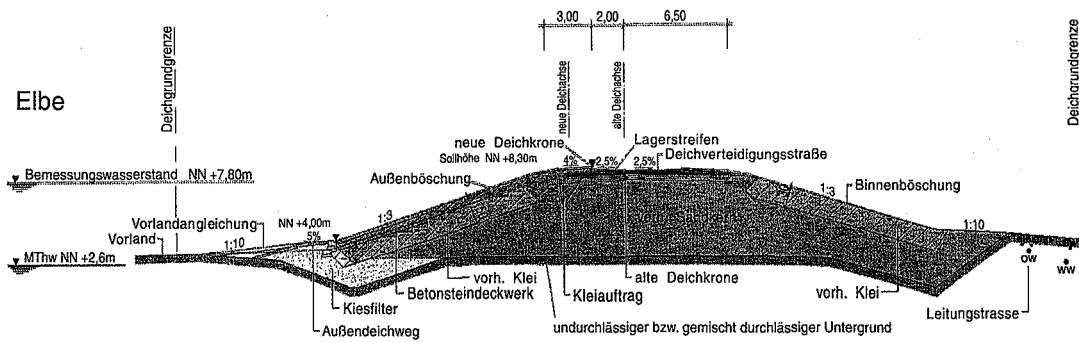
Beispiel 10: Neuengammer Hauptdeich
