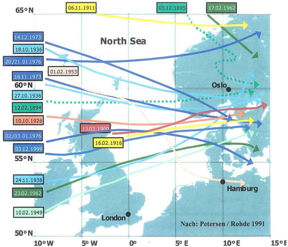
Abb. A 2.3: Zugbahn der Nordsee-Orkantiefs (nach PETERSEN u. ROHDE, 1991)
