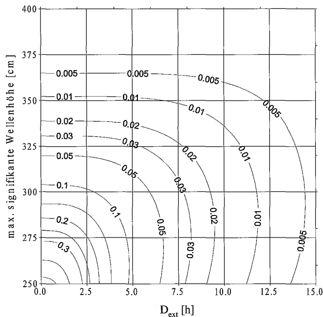
Abb. A 8.8: Gemeinsame Überschreitungswahrscheinlichkeit der Dauer ( D_{\text{ext}} ) und der maximalen signifikanten Wellenhöhe ( H_{m0,\text{max}} ) innerhalb eines Extremereignisses (Daten Heiligenhafen, Ostsee) (Kombinierte univariate Methode, Vergleichswellenhöhe für die Berechnung der Dauer H_{m0,\text{vgl}} = 2,46 \hat{=} 1\text{-jährliche Wellenhöhe} )
