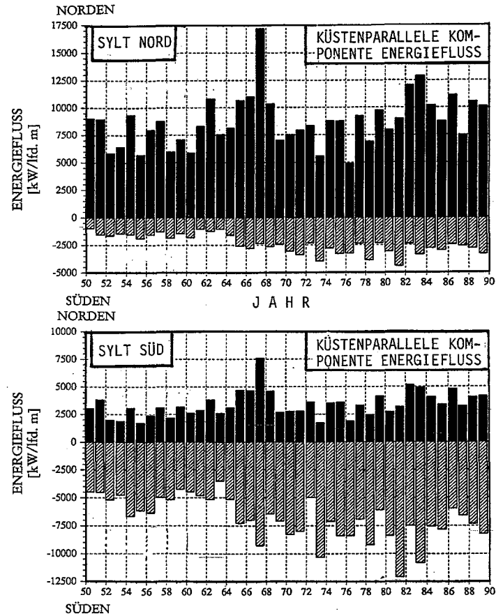
Abb. A 6.11: Rechnerische Ermittlung der küstenparallelen Komponente des jährlichen Energieflusses im Zeitraum 1950 bis 1990 aufgrund von Winddaten und Wind-Wellen-Korrelation (DETTE, 2001), hier für den Nord- und Südteil der Insel Sylt
