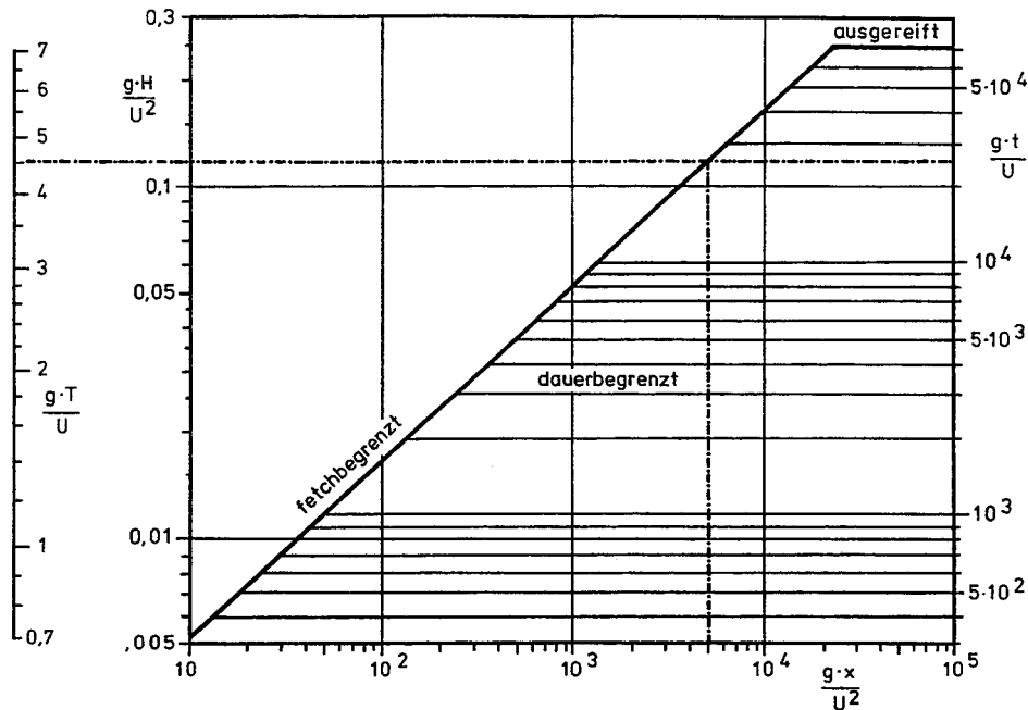
Abb. A 3.39: Dimensionslose Darstellung von fetch- und dauerbegrenztem Windseegang (RICHTER, 1979)
