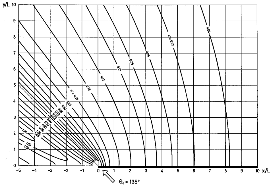
Abb. A 3.31: Diffraction regelmäßiger Wellen an halbinendlichen, totalreflektierenden senkrechten Wänden, SOMMERFELDSche Theorie, Beispiel aus DAEMRICH u. KOHLHASE (1978)
