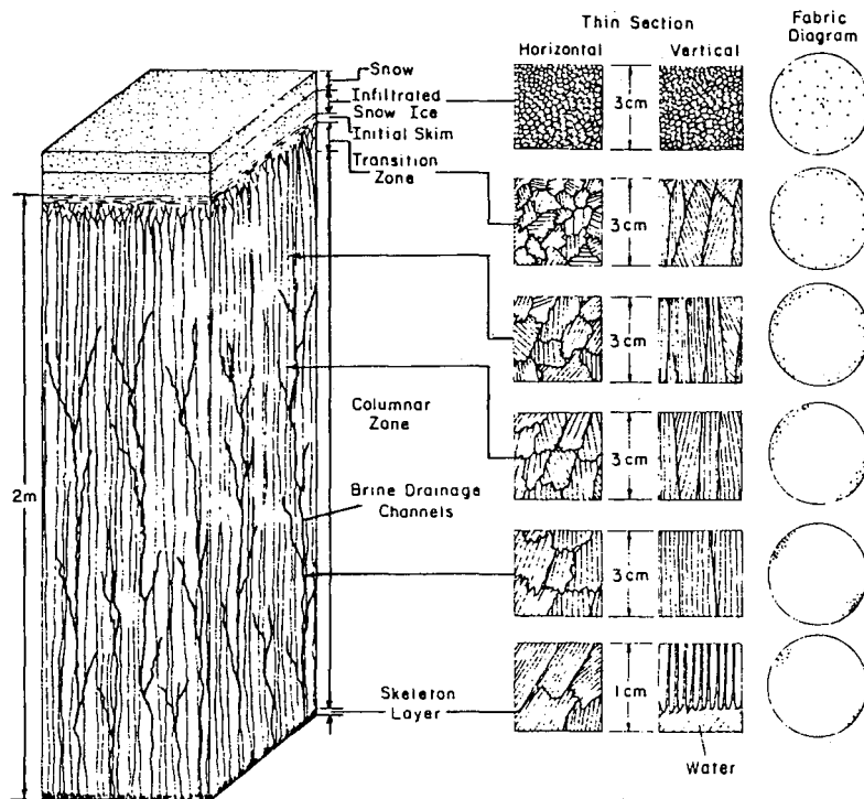
Abb. A 7.3: Schematische Darstellung mit den verschiedenen Schichten von einjährigem Meer-Eis (nach SCHWARZ u. WEEKS, 1977)
