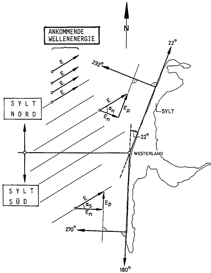
Abb. A 6.11: Rechnerische Ermittlung der küstenparallelen Komponente des jährlichen Energieflusses im Zeitraum 1950 bis 1990 aufgrund von Winddaten und Wind-Wellen-Korrelation (DETTE, 2001), hier für den Nord- und Südteil der Insel Sylt
