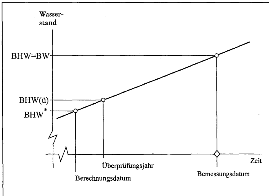
Abb. A. 2.2: Skizze zu den in Kap. 2.1.3 vorgestellten Bemessungswasserständen und zugeordneten Zeitbegriffen
