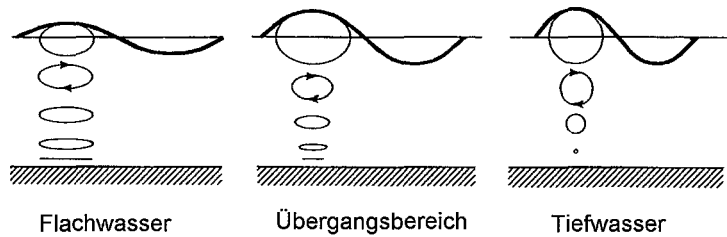
Abb. A 3.6: Erläuterung der Orbitalbewegung oben: Teilchenbahnen an der Oberfläche einer fortschreitenden, harmonischen Welle unten: Veränderung der Orbitalbahnen beim Einlaufen in flaches Wasser
