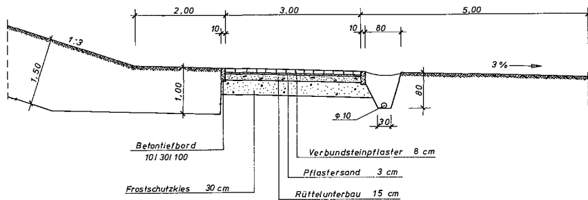
Deichverteidigungsweg im Bereich ohne Bebauung
