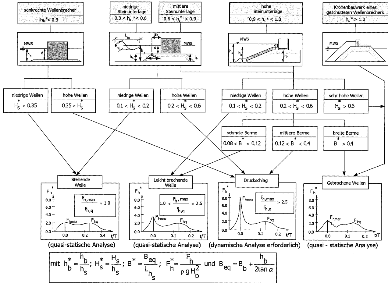
Abb. A 4.3.3. Klassifizierung der Lastfälle nach OUMERACI et al. (2001a)
