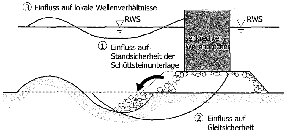
Abb. A 4.3.9: Einfluss der Kolkbildung auf die Standsicherheit der Schüttsteinunterlage und des Betonbauwerkes
