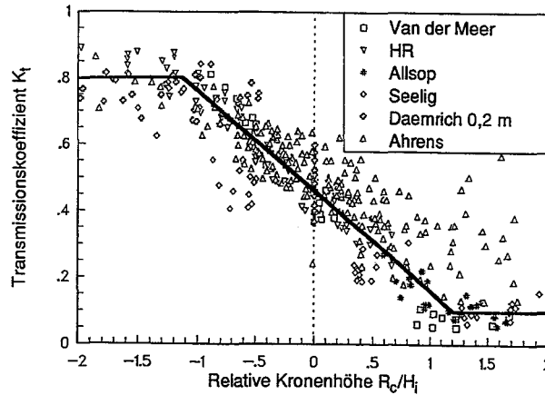
Abb. A 3.36: Wellenmission an Schüttsteinwellenbrechern mit niedriger Kronenhöhe (VAN DER MEER u. D'ANGREMOND, 1991)
