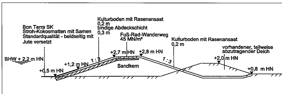
Abb. G 9: Boddendeich Middelhagen, Rügen (Mecklenburg-Vorpommern)
