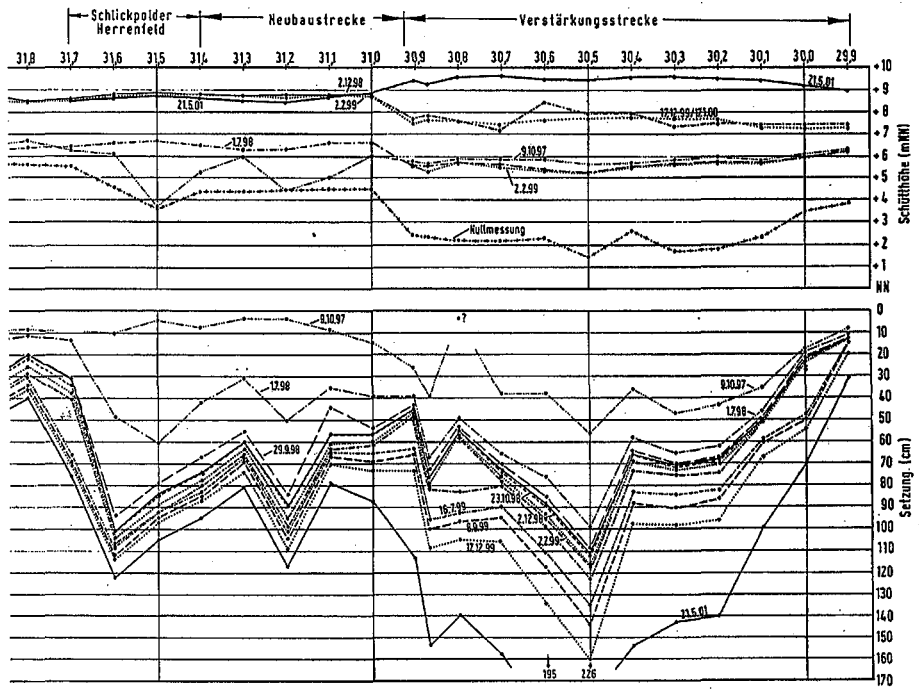
Abb. B 14: Schütthöhen und Setzungen entlang der Deichtrasse Glückstadt-Süd
