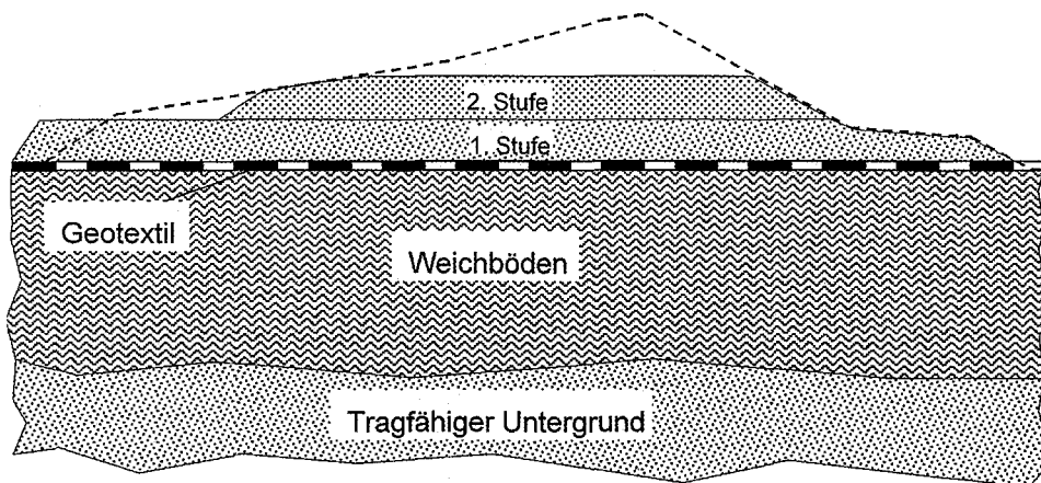
Abb. G 40: Schematische Vorbelastung
