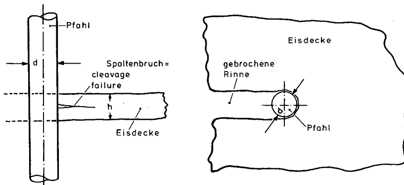
Abb. A 7.11: Spaltbruchversagen der Eisdecke
