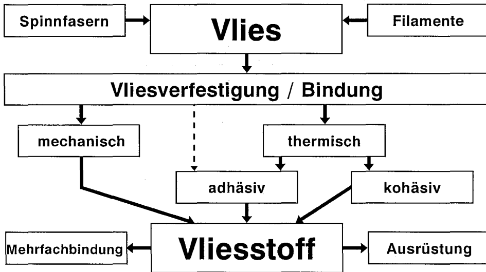
Abb. C 10: Verfestigung/Bindung von Vliesstoffen (SAATHOFF u. ZITSCHER, 2001)
