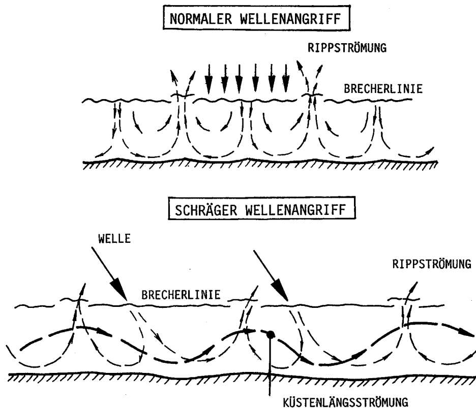
Abb. A 6.1: Ausbildung (schematisch) einer symmetrischen Zellenstruktur der Strömung sowie einer Rippströmung bei küstennormaler Wellenanlafrichtung (oben), mäandrierender Küstenlängsströmung sowie Rippströmung bei schräger Wellenanlafrichtung (unten).
