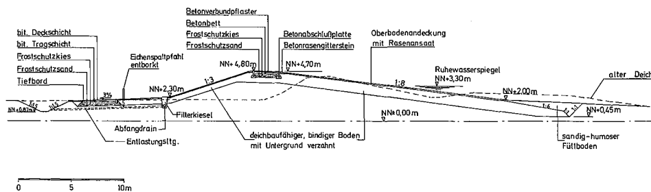
Deichprofil in der nördlichen Ortsrandlage von Grömitz; (Deichverstärkung, 2. Bauabschnitt, 1998)
