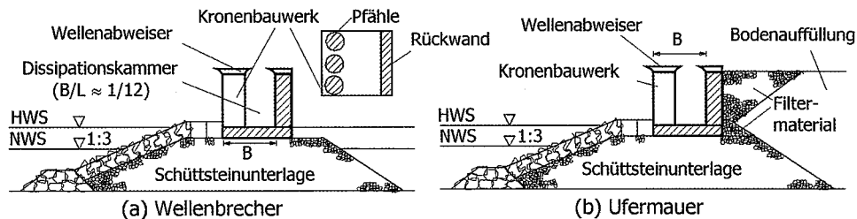
Abb. A 4.3.8: HMCB-Konzept mit Dissipationskammer als Wellenbrecher bzw. Ufermauer
