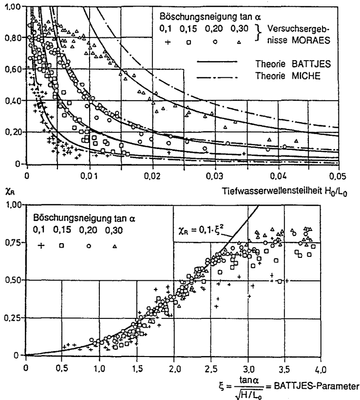
Abb. A 3.29: Reflexion an glatten Böschungen (BATTJES, 1974)
