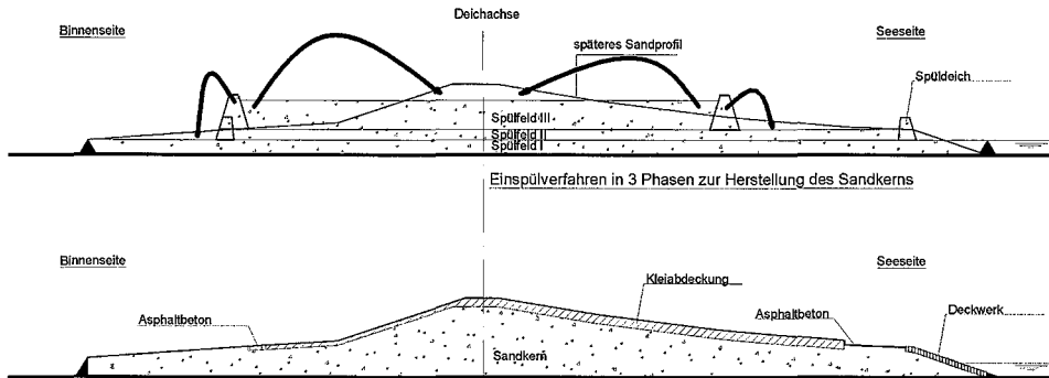
Abb. G 46: Neubau eines Seedeiches mit in drei Spülfeldebene eingespültem Sandkern
