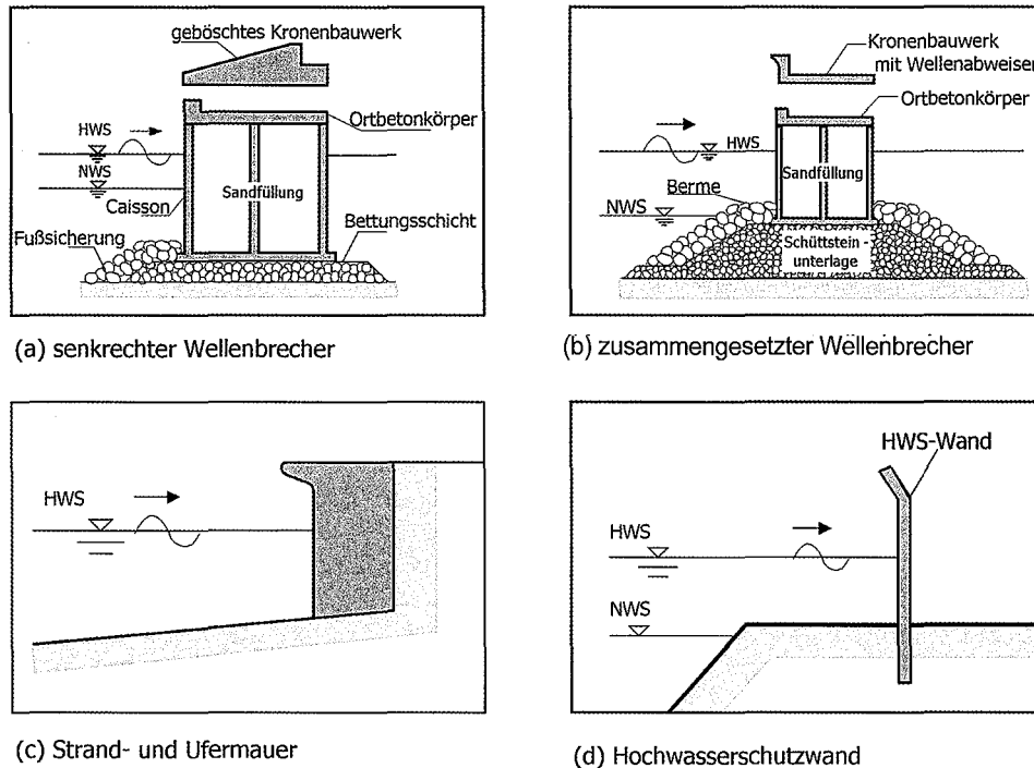
Abb. A 4.3.1: Ausgewählte Bauweisen von senkrechten Wellenschutzbauwerken (schematisch)
