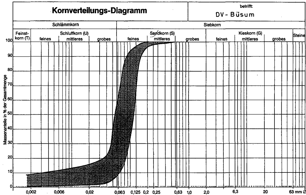
Abb. G 19: Variationsbreite der Korngrößenverteilung eines kleiligen Wattsandes in der Sandentnahme Büsum-Augustenhof
