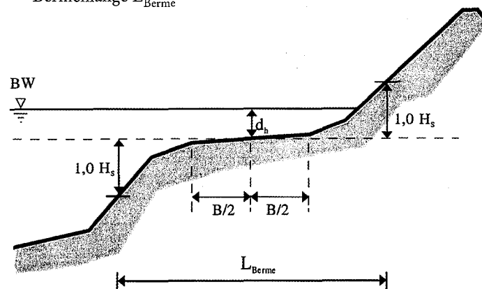
Abb. A 4.2.10: Berücksichtigung einer Berme im Deichquerschnitt bei der Ermittlung der Deichneigung \alpha und der wirksamen Bermenlänge L_{\text{Berme}}
