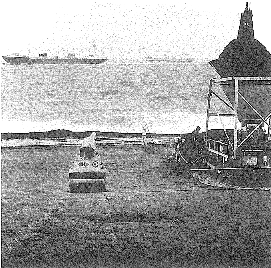
Abb. G 49b: Raupengeführter Vertikalfertiger im Einsatz (CUR, 1995)
