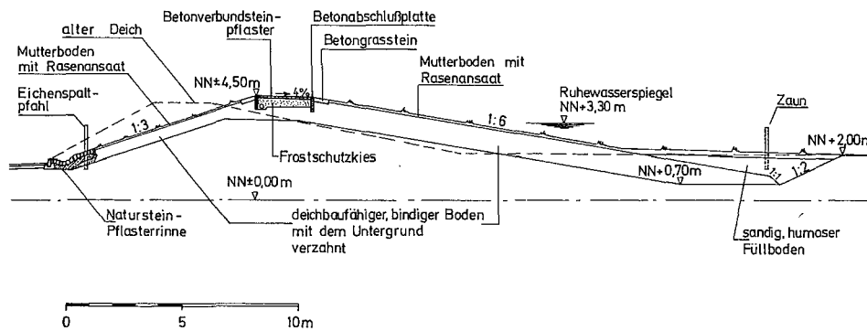
Deichprofil in der Ortslage von Grömitz; (Deichverstärkung, 1. Bauabschnitt, 1990/92)
