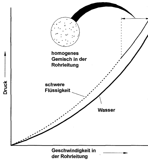
Abb. G 43: Mit steigender Fließgeschwindigkeit des Wassers nimmt der Druckverlust pro Längeneinheit zu (BRAY et al., 1997)
