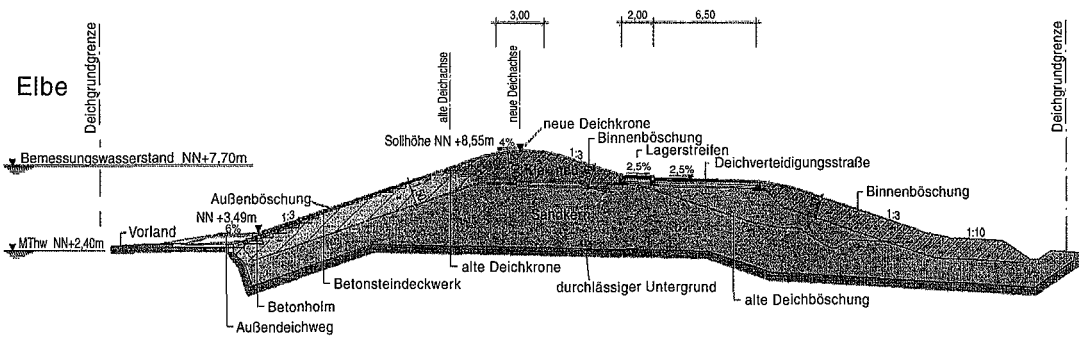
Beispiel 9: Zollenspieker Hauptdeich
