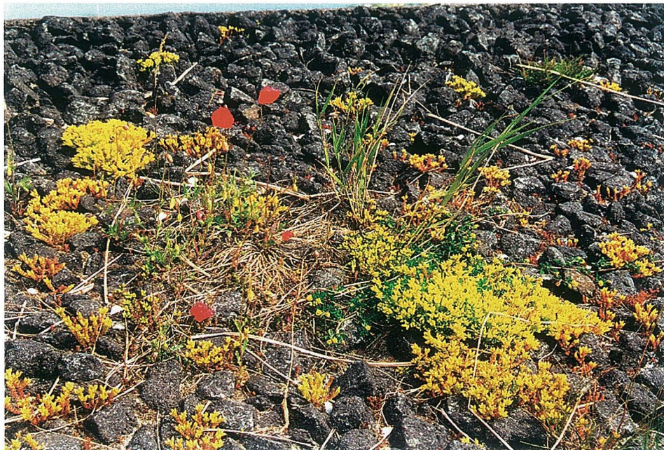
Abb. G 51b: Deichverstärkung Tümlauer Koog 1994/95 (Westabschnitt), Stat. 2+660 bis Stat. 2+860: Deckwerk aus 20 cm Mastixschotter auf der Außenböschung bis zur Dammkrone – wasserdurchlässig und begrünt
