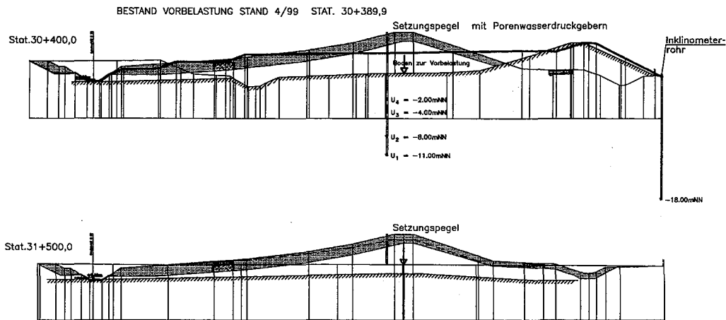
Abb. B 13: Charakteristische Deichquerschnitte
