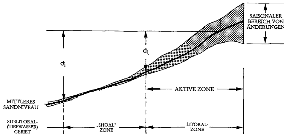
Abb. A 6.6: Aufteilung des Unterwasserprofils im Küstenvorfeld auf der Grundlage von Grenztiefen („closure depths“), hier: d_1 als Grenze, bis zu der sich jahreszeitliche oder saisonale Änderungen des Ober- und Unterwasserstrandprofils in beachtlichen Größenordnungen abspielen und d_i als Grenze, wo das mittlere jährliche Wellenklima noch eine Sedimentbewegung bewirkt (HALLERMEIER, 1981)
