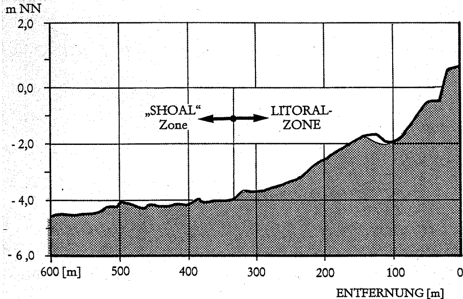
Abb. A 6.7: Veranschaulichung des Überganges von der Litoral- zur „Shoal“-Zone (Grenztiefe d_l ) am Beispiel eines Unterwasserstrandprofils der Ostsee
