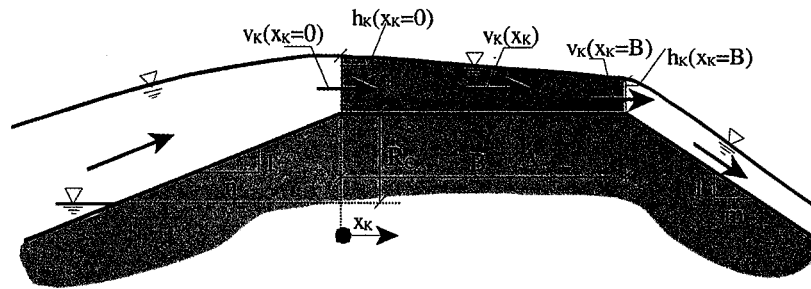
(b) Definition der Strömungsgrößen auf der Deichbinnenböschung
