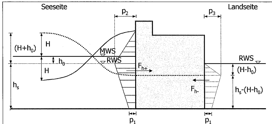
Tafel A 4.3.3: Druckbelastung durch stehende Wellen (Verfahren nach SAINFLOU und Hinweise auf das Verfahren von MICHE-RUNDGREN)
