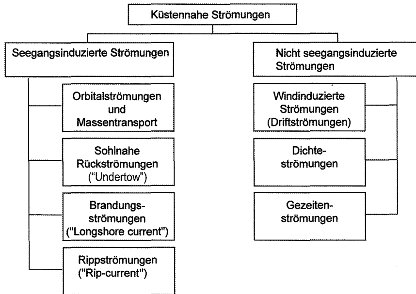
Abb. A 5.1: Küstennahe Strömungen
