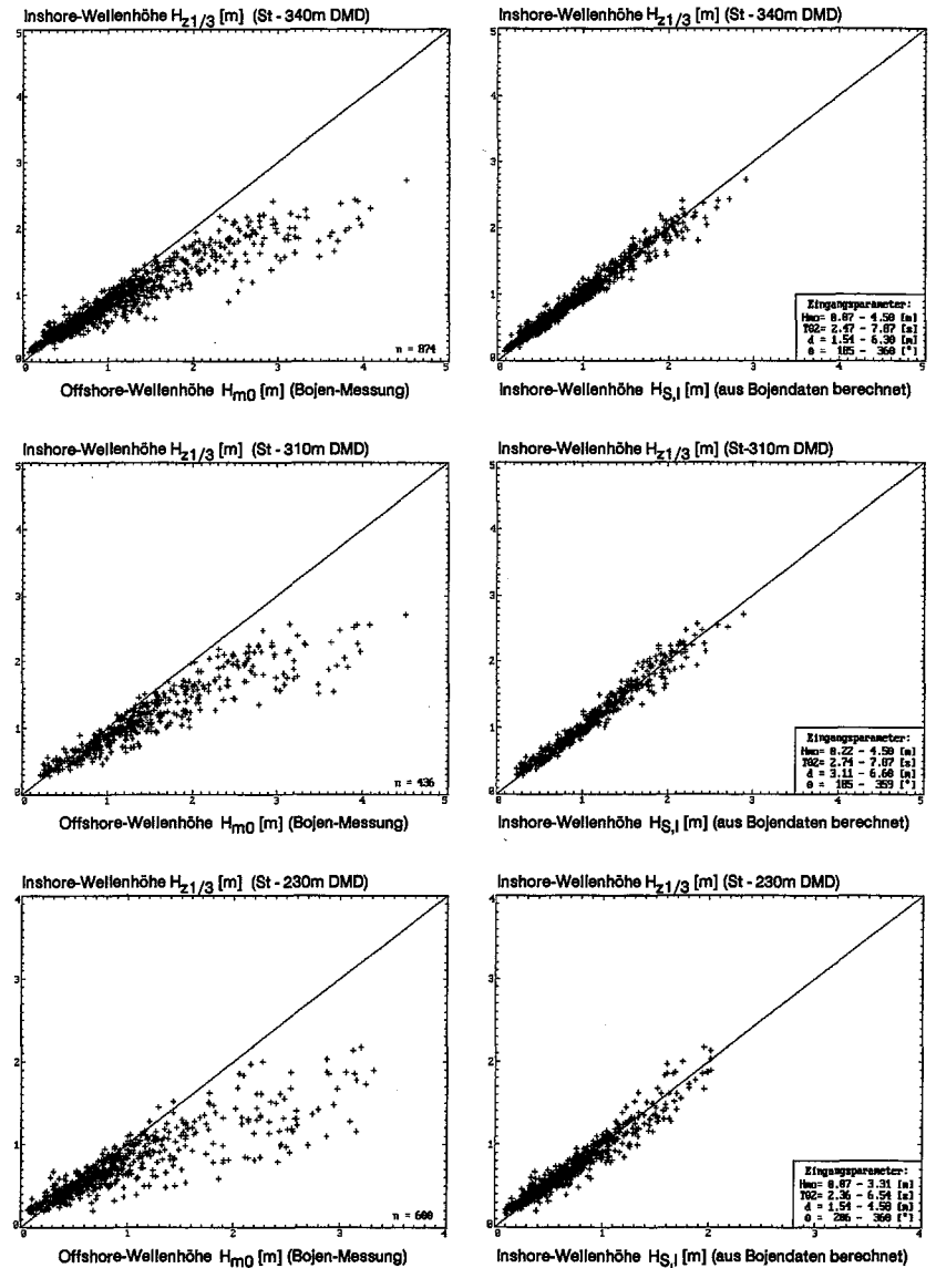
Abb. A 3.37: Wellentransmission an einem Brandungsriff, Beispiel Sylt (STROTMANN u. KOHLHASE, 1991); links: Sohllagen im Profil Rantum und Lage der ausgewerteten Messstationen; rechts: Vergleich der an den Druckmessdosen (DMD) gemessenen Offshore-Wellenhöhen (a) und Verifikation des theoretischen Ansatzes (b) durch Variation der kritischen Wellenhöhe auf dem Riff
