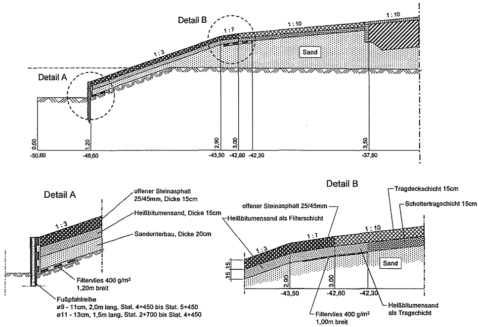
Abb. G 50a: Deichverstärkung Friedrich-Wilhelm-Lübke-Koog hinter Vorland: Fußdeckwerk 2001/2002 aus 15 cm Mastixschotter auf 15 cm Bitumensand-Filter bis zur Überslaggsicherung
