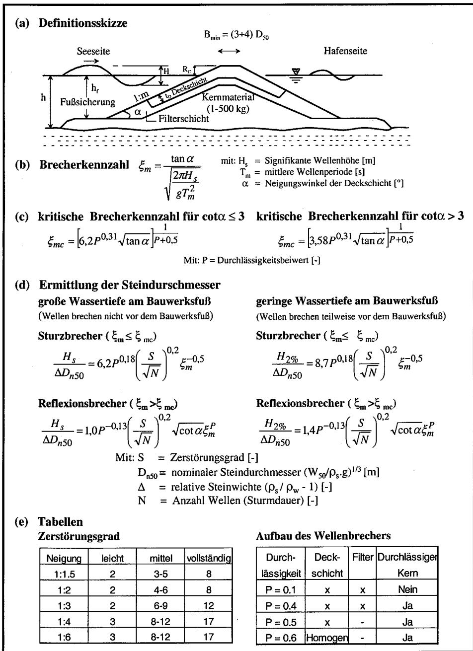
Abb. A 4.2.15: Bemessungsformeln für geschüttete Wellenbrecher – VAN DER MEER-Formel – (VAN DER MEER, 1985; 1998)
