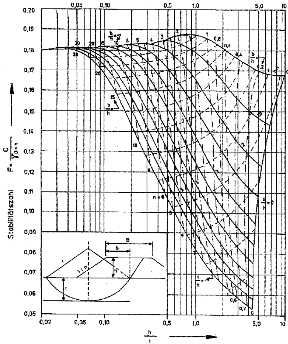
Abb. B 7: Standsicherheitsabschätzung für den Bauzustand nach SIEDEK, GRASSHOFF, KÜBLER (1969)
