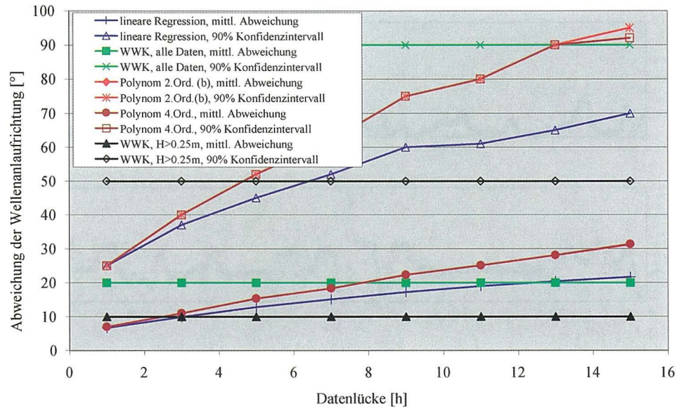
Abb. A 3.53: Abweichung von berechneten Wellenaufrichtungen von Messwerten für ausgewählte Verfahren zur Schließung von Datenlücken (a): Messwert vor und nach der Datenlücke; (b): Einbeziehung mehrerer Messwerte vor und nach der Datenlücke
