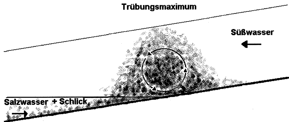
Abb. A 5.6: Salzkeileffekt (nach WELLERSHAUS, 1982)
