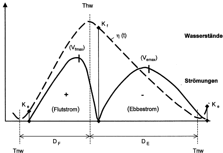
Abb. A 5.5: Parameter zur Beschreibung der Tide
