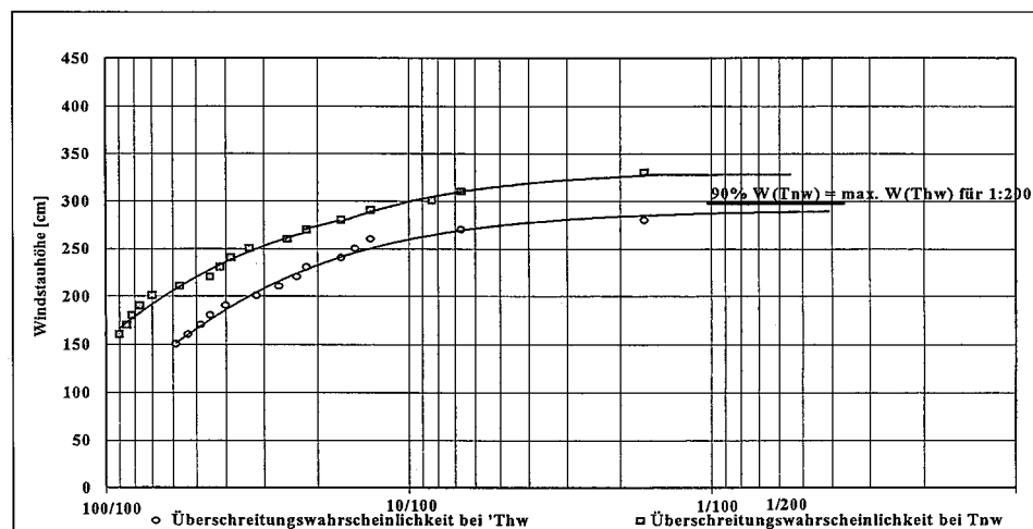
Abb. A 2.9. Überschreitungswahrscheinlichkeit der Windstauhöhen auf Norderney für die Jahre 1938-1997 (GÖNNERT u. SIEFERT, 1998)
