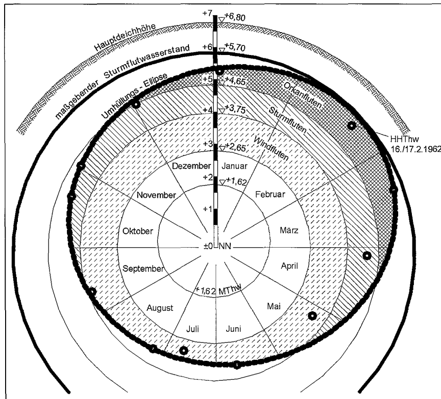
Abb. G 67: Monatsrose der Sturmzeiten am Beispiel der über 100-jährigen Beobachtungszeitspanne des Pegels Wilhelmshaven mit
