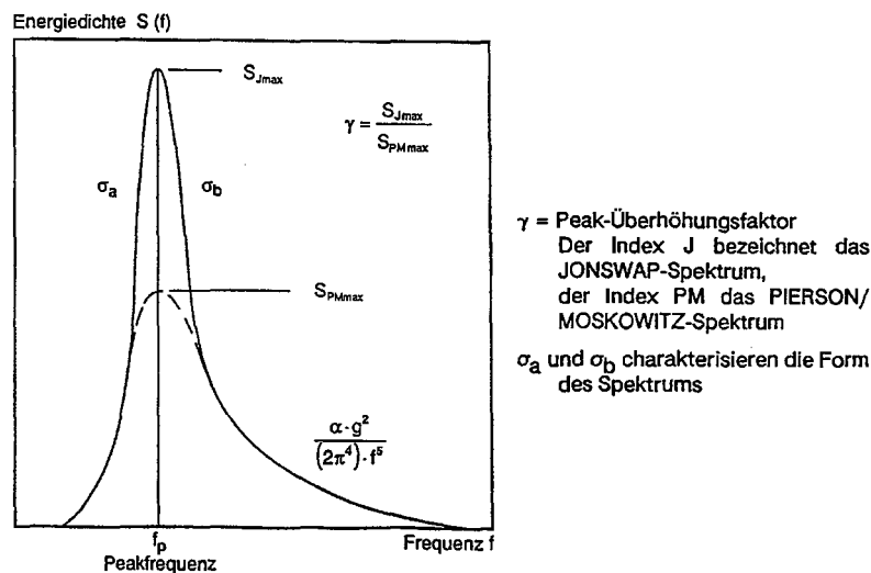
Abb. A 3.13: Formen von Tiefwasserseegangsspektren und Bezeichnungen (RICHTER, 1981)
