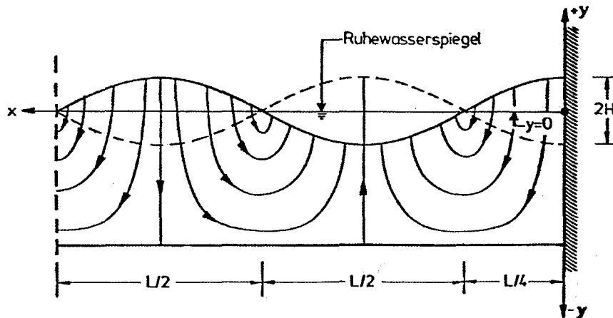
Abb. A 5.9: Schematisches Stromlinienbild einer stehenden Welle
