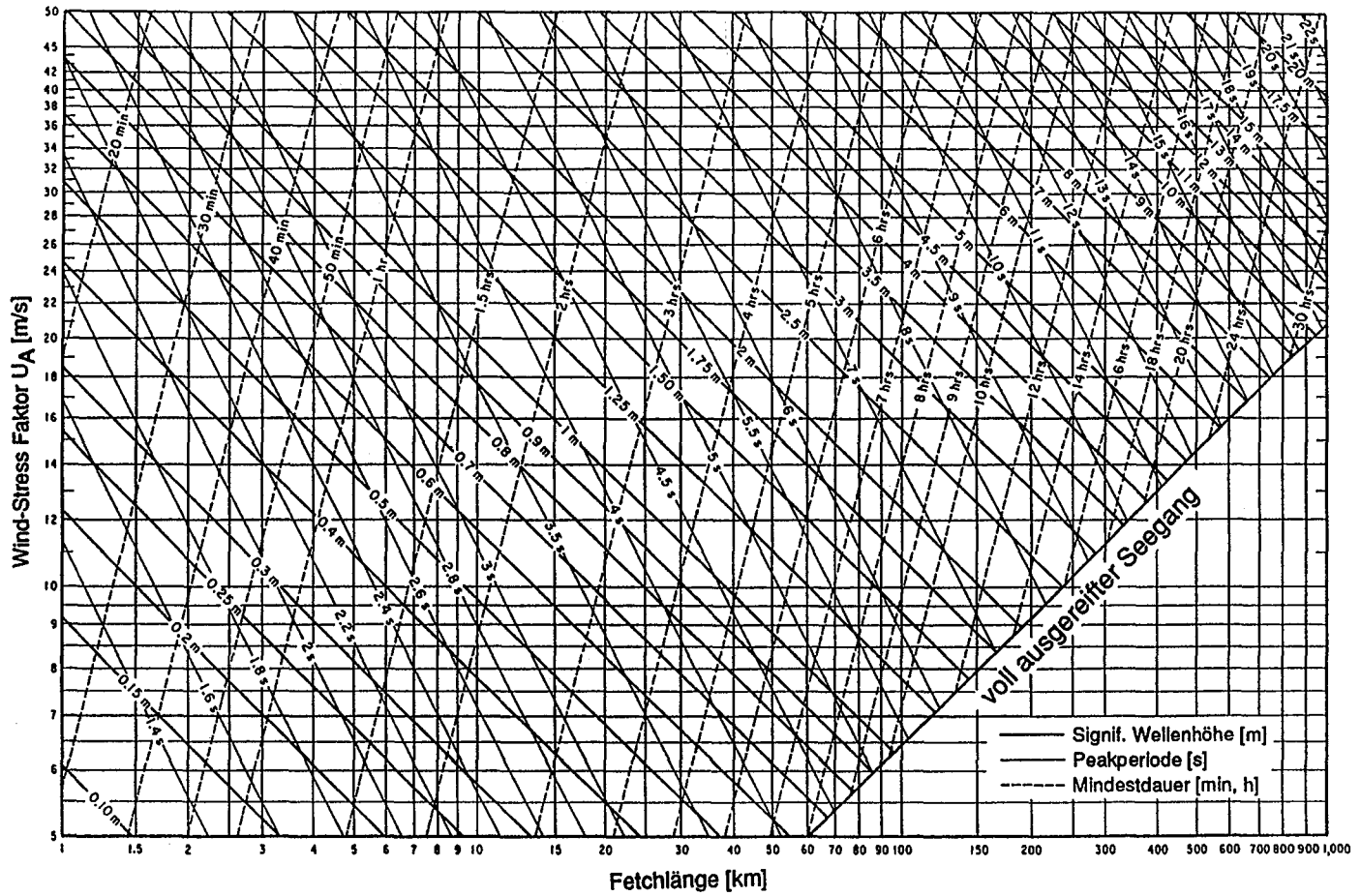
Abb. A 3.40: Seegangsvorhersage nach SPM für Tiefwasserbedingungen (CERC, 1984)
