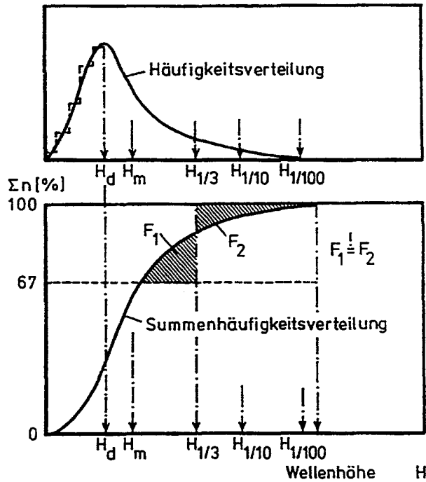
Abb. A 3.11: Prinzip der Auswertung von Zeitbereichparametern aus einer Häufigkeitsdarstellung (Histogramm) ( H_d ist hier die „dominante“ Welle und nicht zu verwechseln mit dem im Folgenden verwendeten Index d für downcrossing)
