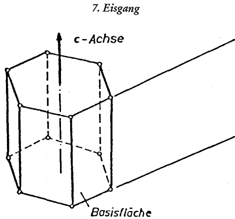
Abb. A 7.2: Vereinfachtes Modell eines hexagonalen Kristallgitters
