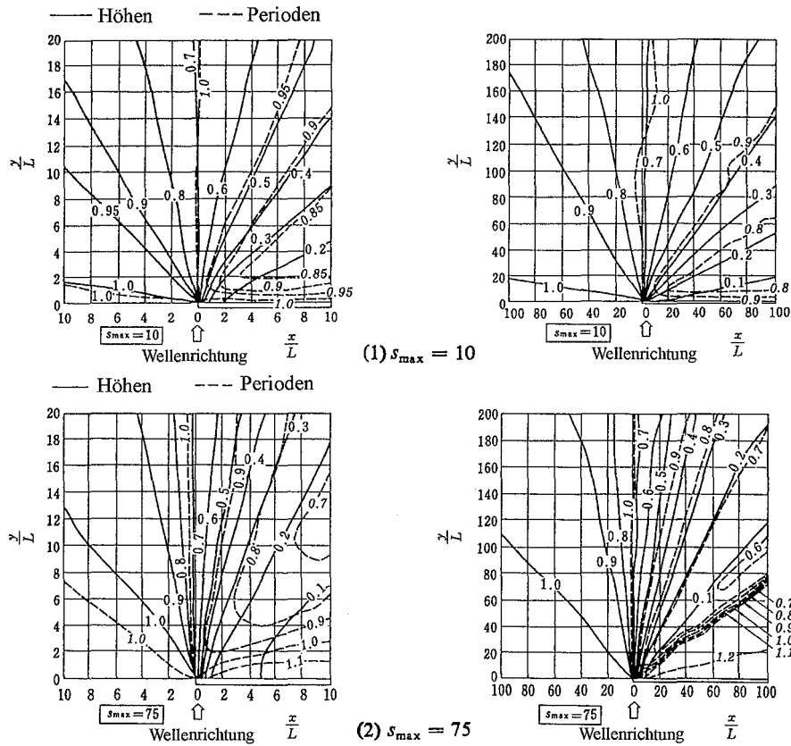
Abb. A 3.33: Diffraction von Seegangsspektren, halboundlicher Wellenbrecher (CERC, 1984)
