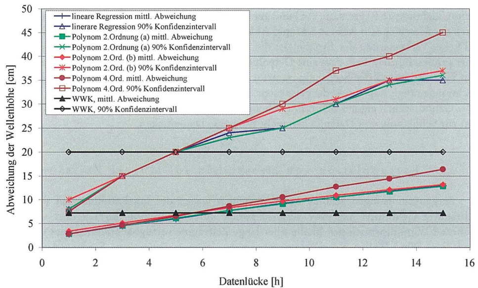
Abb. A 3.52: Abweichung von berechneten Wellenhöhen von Messwerten für ausgewählte Verfahren zur Schließung von Datenlücken (a): Messwert vor und nach der Datenlücke; (b): Einbeziehung mehrerer Messwerte vor und nach der Datenlücke
