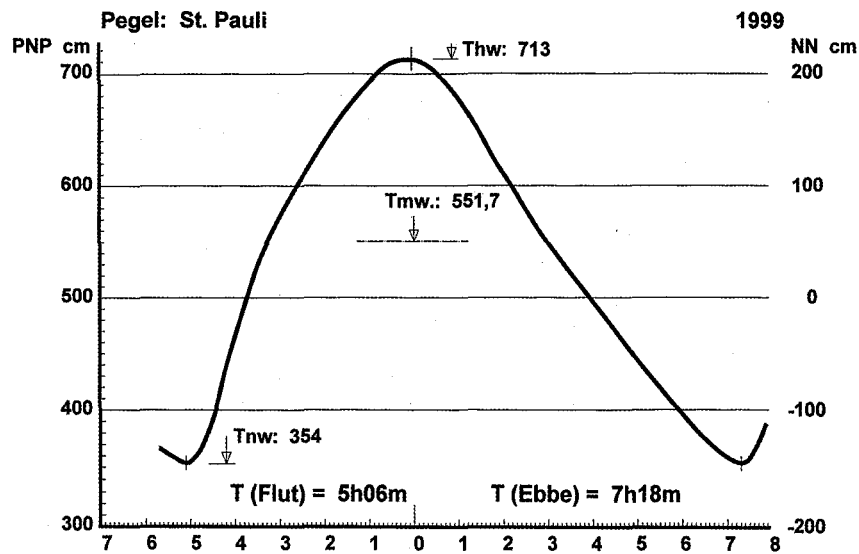
Abb. A 5.4: mittlere Tidekurve am Pegel St. Pauli
