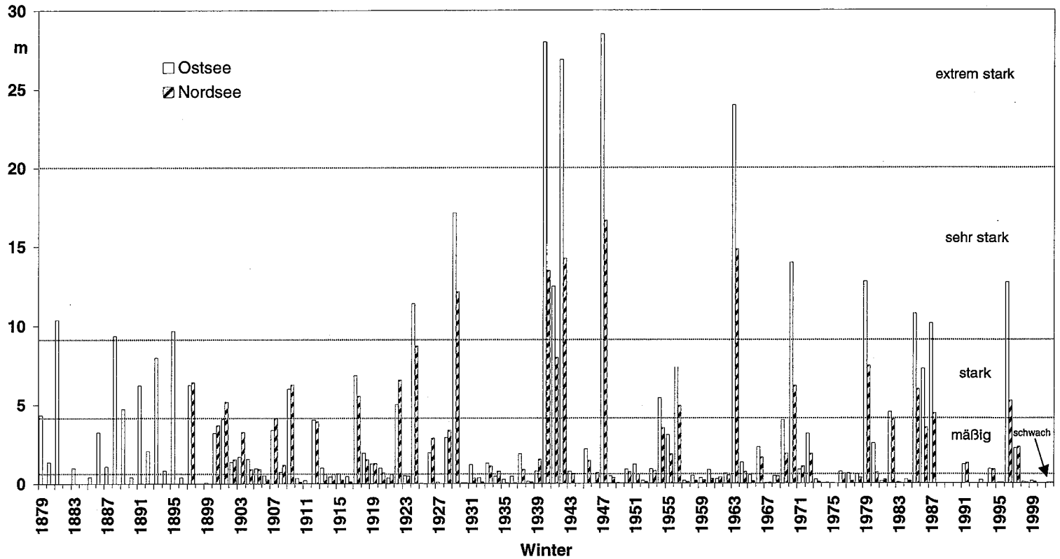
Abb. A 7.13: Die flächenbezogene Eisvolumensumme der deutschen Nordseeküste von 1897–2001 und der deutschen Ostseeküste von 1879–2001 (1946 keine Daten). Die horizontalen punktierten Linien gelten nur für die Eiswintertypen der deutschen Ostseeküste
