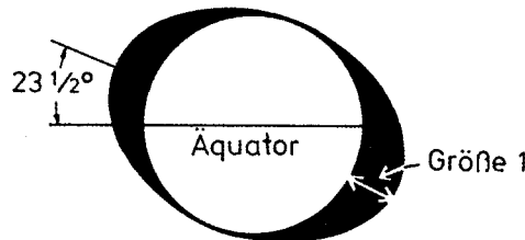
Abb. A 5.2: Wirkungen des Mondes und der Sonne auf die Wasseroberfläche
