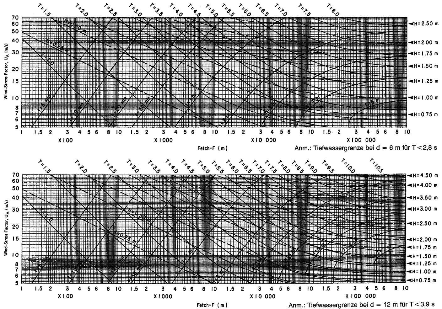
Abb. A 3.41: Seegangsvorhersage nach dem SPM für Flachwasserbedingungen (CERC, 1984); oben: Wassertiefe d = 6 m; unten: Wassertiefe d = 12 m
