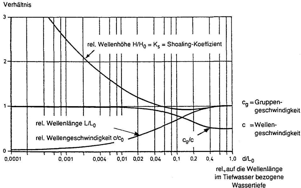
Abb. A 3.17: Wellenverformung bei abnehmender Wassertiefe (Shoaling), lineare Theorie
