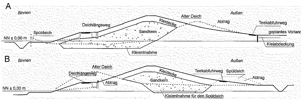
Abb. G 47 A + B: Deichverstärkung je nach verfügbarer Fläche:
