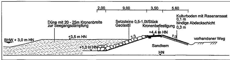
Abb. G 6: Seedeich Boltenhagen-Tarnowitz mit leichtem Setzdeckwerk (Mecklenburg-Vorpommern)
