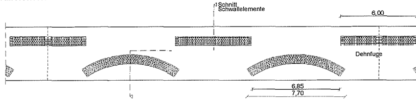
Lageplan Schwallelemente
