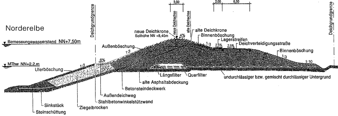
Beispiel 8: Gauerter Hauptdeich
