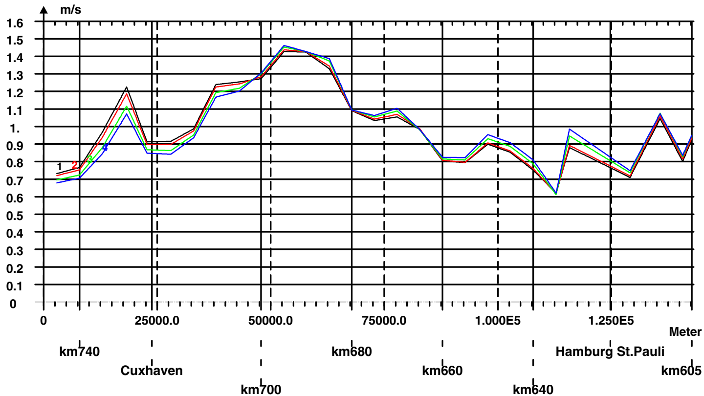
Bild 25: Maximalen Ebbestromgeschwindigkeit (querschnittsgemittelt) für die Sturmflutszenarien SF76 ohne slr (as01), slr+25 cm (as02), slr+80 cm (as04) und slr+115 cm (as05) entlang des Elbefahrwassers von Elbe-km 745 bis Elbe-km 605.
