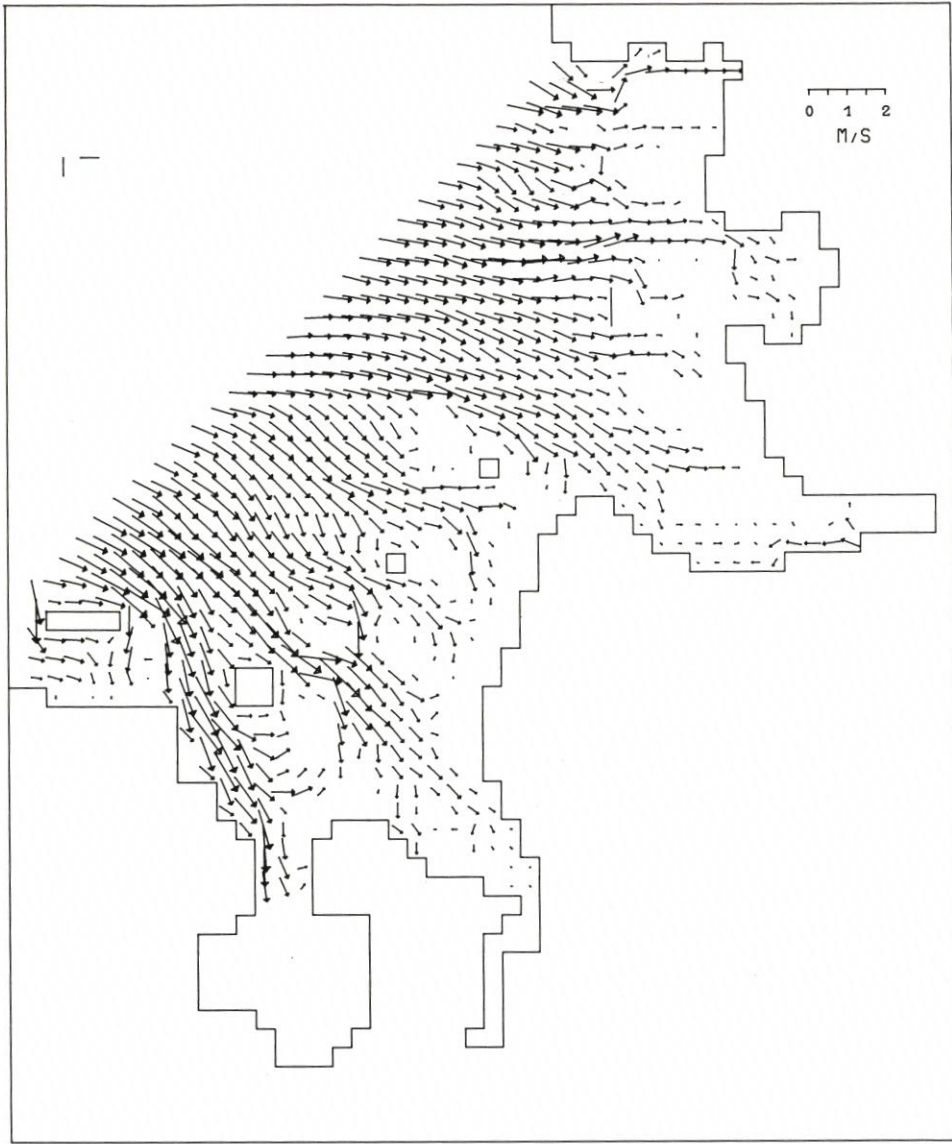
Abb. 20. Regionalmodell „Innere Deutsche Bucht“ – Strömungsverteilung bei auflaufend Wasser (8. 7. 1976, 18.00 h , etwa halbe Tide)
