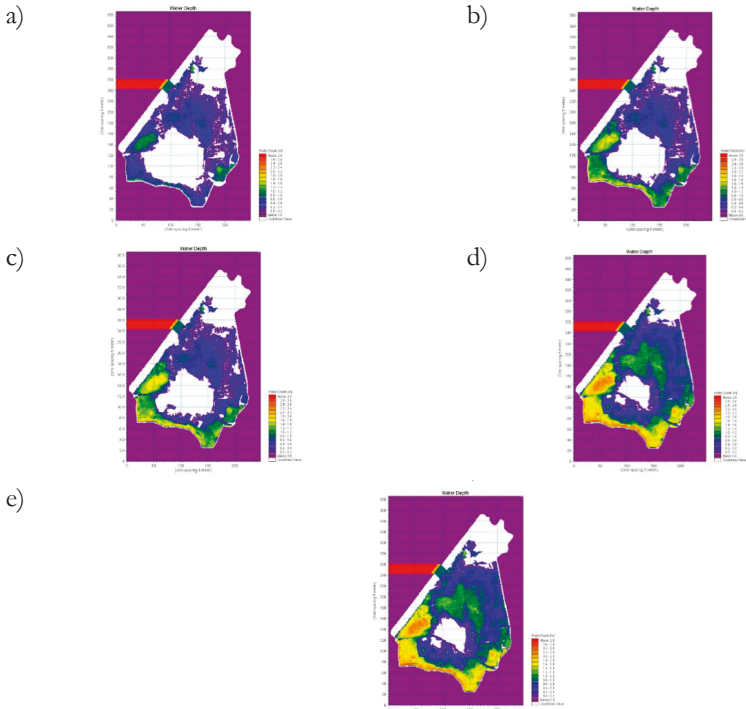
Abbildung 27: Maximale Überflutungsflächen a) k_{St} = 5 \text{ m}^{1/3}/\text{s} , b) k_{St} = 10 \text{ m}^{1/3}/\text{s} , c) k_{St} = 15 \text{ m}^{1/3}/\text{s} , d) k_{St} = 25 \text{ m}^{1/3}/\text{s} und e) k_{St} = 32 \text{ m}^{1/3}/\text{s} .
