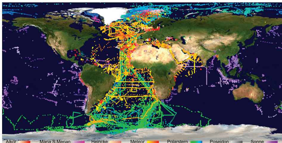
Abbildung 1: Aktueller Status der Probennahmestationen und Fahrten der wichtigsten deutschen Forschungsschiffe (Quelle PANGAEA 2013).
