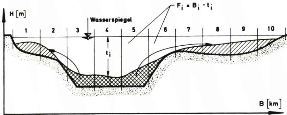
Abb. 3. Durchflußquerschnitt, schematisch
