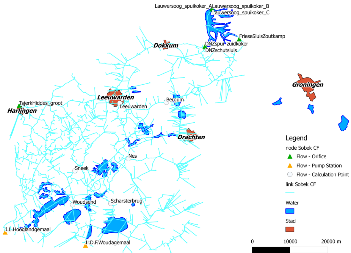
Abbildung 1: Sobek-Modell des Gewässernetzes im Verbandsgebiet der Wetterskip Fryslân mit den Sielen „Tsjerk Hiddesluis“, „Dokkumer Nieuwe Zijlen“ (DNZ), „Friese Sluis“ und den Schöpfwerken „Hooglandgemaal“ und „Woudage-maal“ (Becker, 2013)
