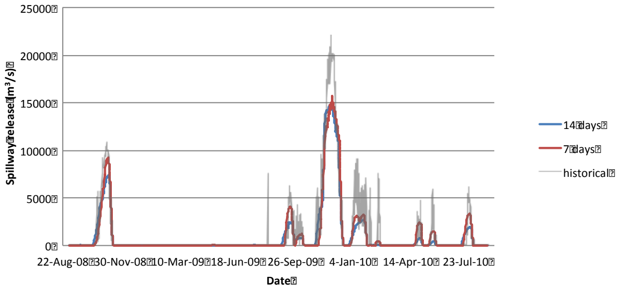
Abbildung 5: Abgabe (release) über die Hochwasserentlastung (spillway) unter Anwendung des Optimierungstools mit 7-Tage und 14-Tage Vorhersage sowie der historischen Steuerung (Schruff, 2011)
