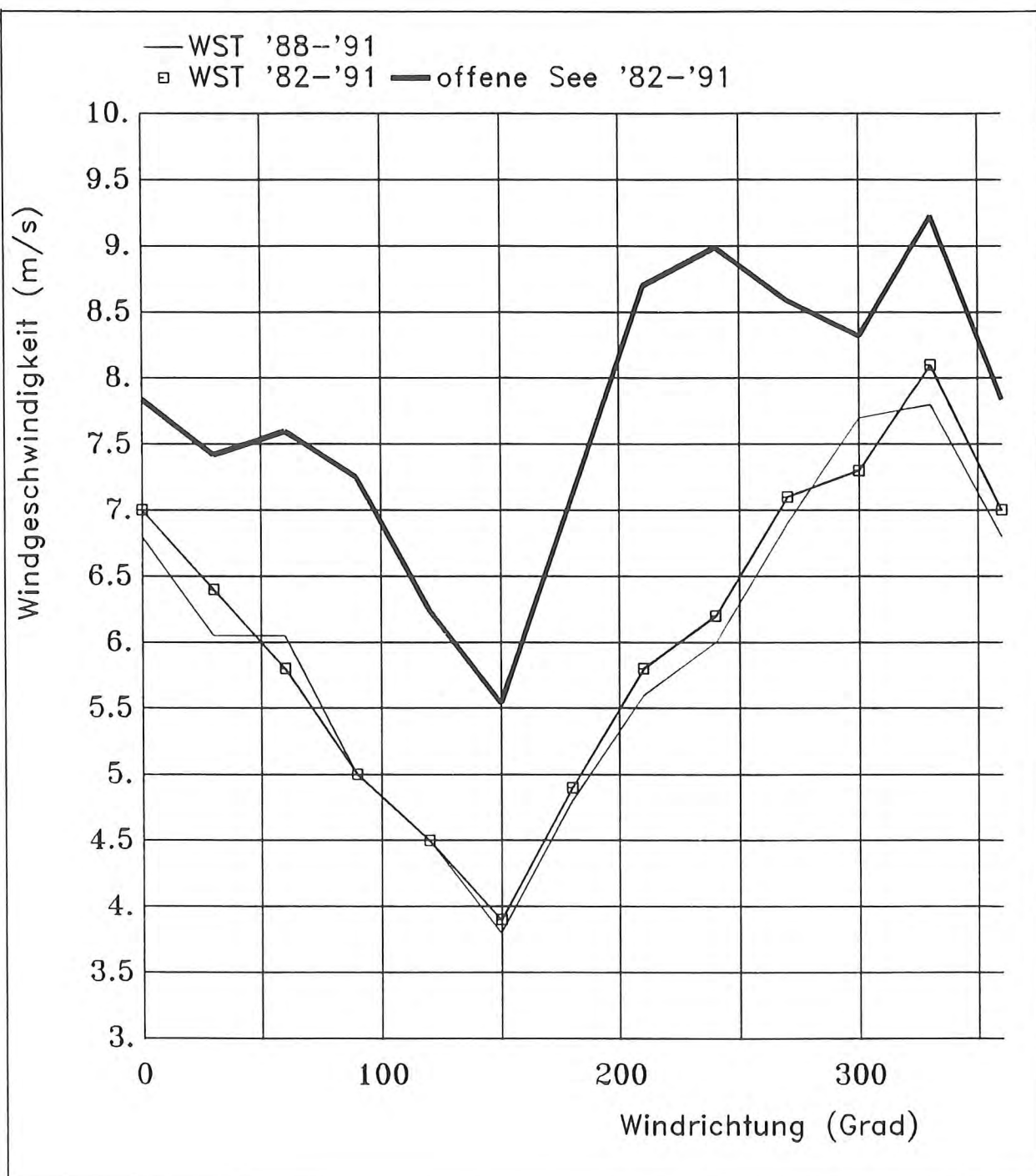
Abbildung 4.4: Richtungsabhängige klimatologische Mittelwerte der Windgeschwindigkeit für die Jahre 1982-1991 an der Wetterstation (WST) und auf der freien See. Zum Vergleich für die Wetterstation auch das Mittel über den Projektzeitraum 1988-1991 (dünne Linie).
