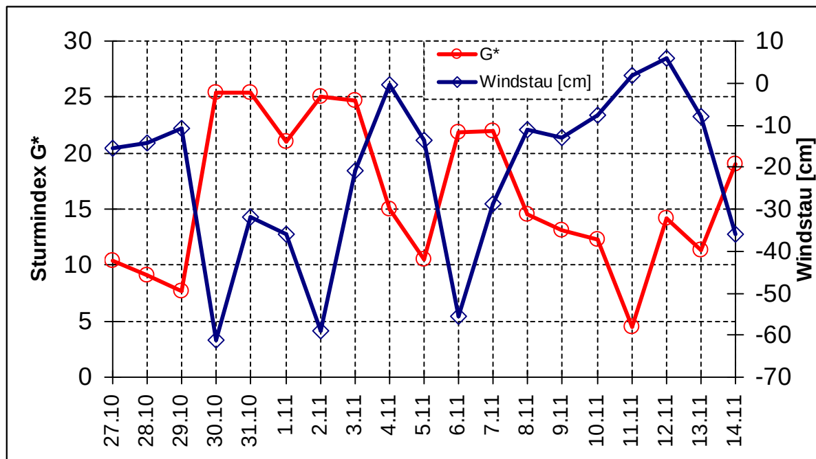
Abbildung 14: Sturminde und potentieller Windstau in der südlichen Ostsee im Zeitraum der Sturmflut aus dem Jahr 1872, berechnet aus dem bodennahen Luftdruckfeld des EMSLP.
