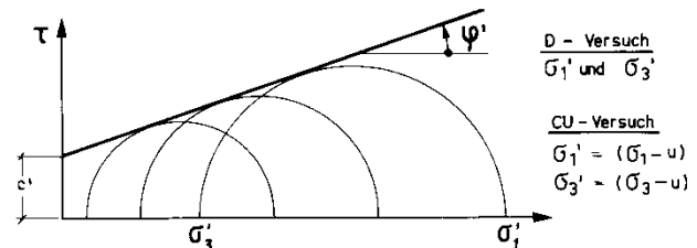
Bild 18: Konsolidierter, dräniertes (D-Versuch) bzw. konsolidierter, undränniertes (CU-Versuch) Versuch aus (Kempfert et al. 1998)
