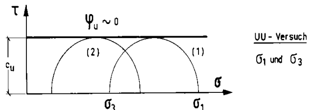
Bild 19: Unkonsolidiertes, undränniertes (UU-Versuch) Versuch aus (Kempfert et al. 1998)
