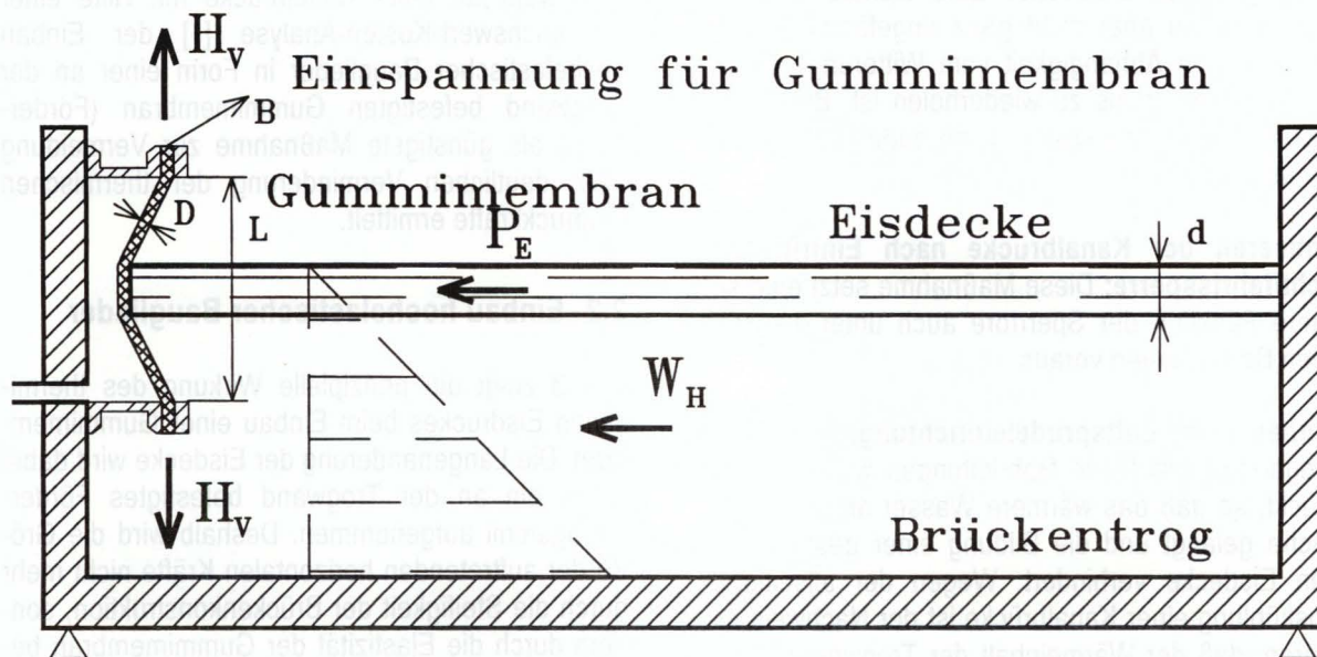
Bild 3: Schematische Darstellung der Wirkung des thermischen Eisdrukkes beim Einbau einer Gummimembran
