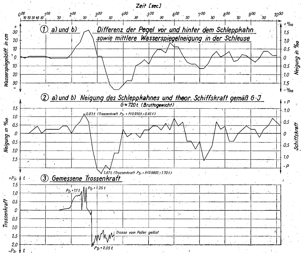
Bild 7 Donaukraftwerk Jochenstein. Zeitlicher Verlauf der Wasserspiegelneigung, der Schiffsneigung und der Trossenkräfte in der Südschleuse während des Abschaltversuches am 8. 6. 1956.
