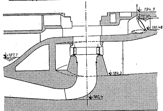
Vorschlag 4: Turbine mit Nebenauslaß als Klappe mit horizontaler Welle
