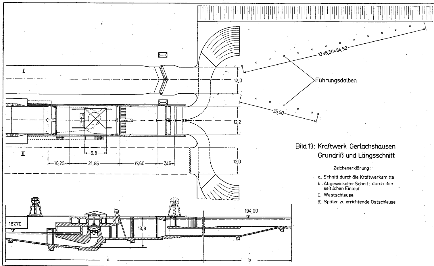
Bild 13 Kraftwerk Gerlachshausen. Grundriß und Längsschnitt.
