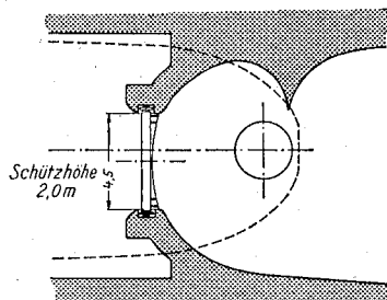
Vorschlag 3: Turbine mit Nebenauslaß als Klappe mit vertikaler Welle
