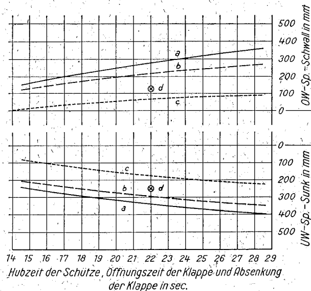
Bild 12 Mainstaustufe Gerlachshausen. Schwall- und Sunkvergleich bei den drei verschiedenen Anordnungen in Abhängigkeit von der Verschlussbewegung in sec.
