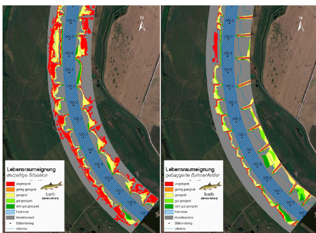
Bild 8: Detail des Pilotgebietes Klöden, mit dem Fischmodell MOFIR 2 modellierte Lebensraumeignung für die adulte Barbe ( Barbus barbus ), links: Ausgangszustand, rechts: Zustand nach Ausbaggerung der Bühnenfelder, beide bezogen auf mittleren Niedrigwasserabfluss
