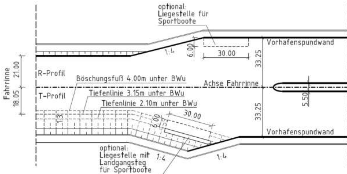
Abb. 7 Übergänge vom Vorhafen einer Doppelschleuse in Spundwandbauweise zur freien Strecke (oben: in Verlängerung eines R-Profils; unten: in Verlängerung eines T-Profils)
