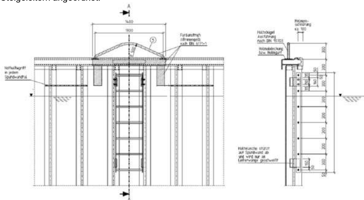
Abb. 11 Anordnung von Steigeleitern an Spundwandliegestellen
