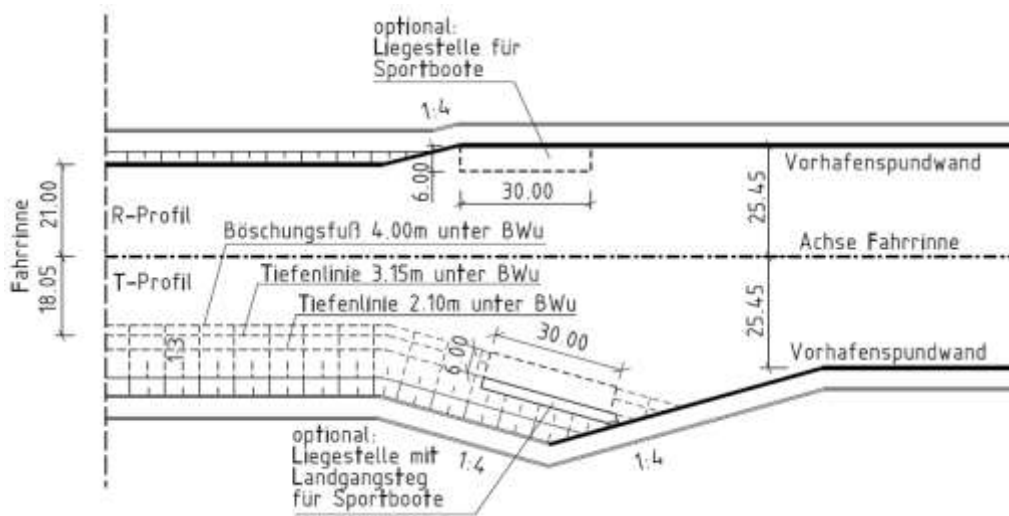
Abb. 6 Übergänge vom Vorhafen einer Einzelschleuse in Spundwandbauweise zur freien Strecke (oben: in Verlängerung eines R-Profils; unten: in Verlängerung eines T-Profils)
