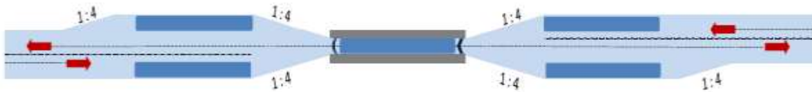
Abb. 2 Verschwenkung der Kanalachse in Vorhäfen einer Einzelschleuse (Prinzip-Skizze)
