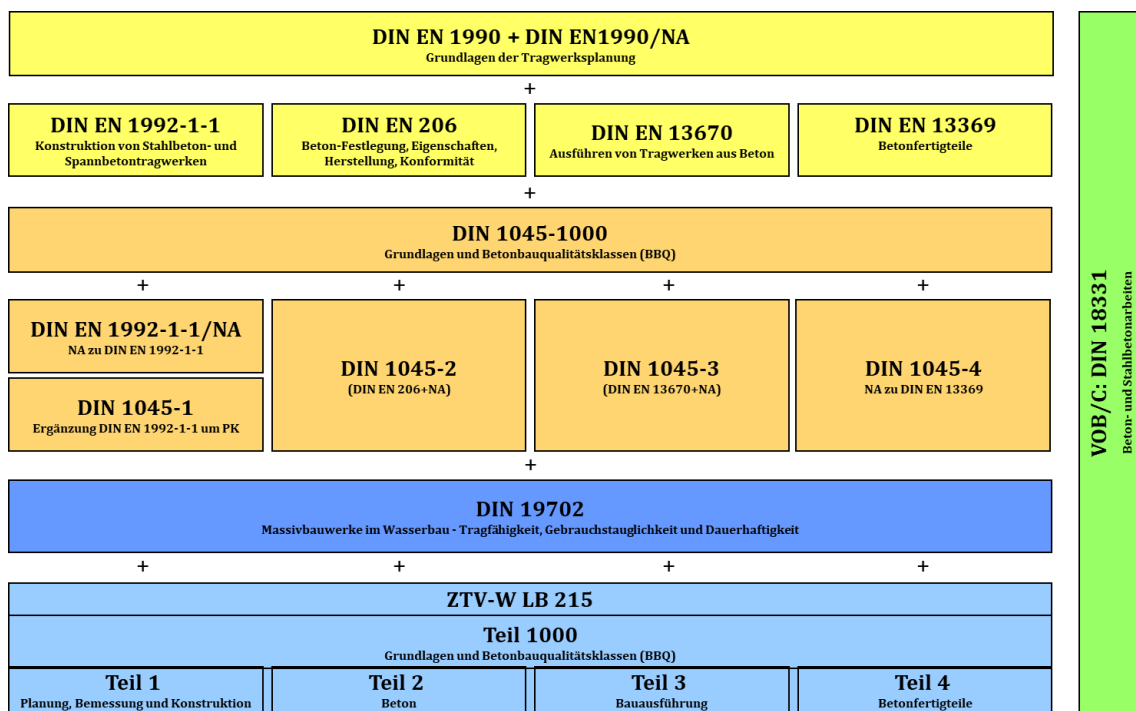
Abbildung 1: Überblick über die maßgebende Normungssituation für ZTV-W LB 215
