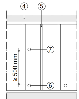
Prinzipskizze 4: Anordnung von elektrischen Einbauteilen in Holztafelbauwänden
