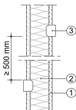
Prinzipskizze 4: Anordnung von elektrischen Einbauteilen in Holztafelbauwänden
